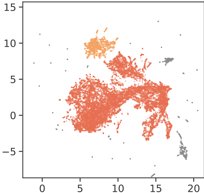
H. halys - UMAP
