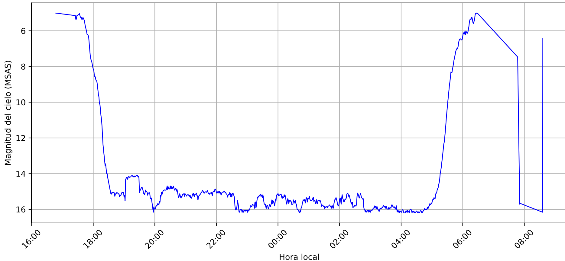
Magnitud del cielo en Usaquén (2026-06-15 16:00:00 a 2026-06-16 10:00:00)
