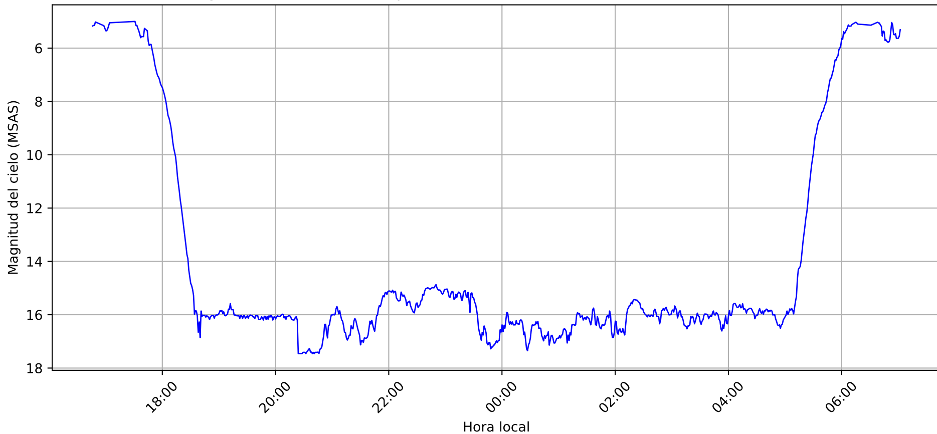
Magnitud del cielo en Usaquén (2026-06-16 16:00:00 a 2026-06-17 10:00:00)
