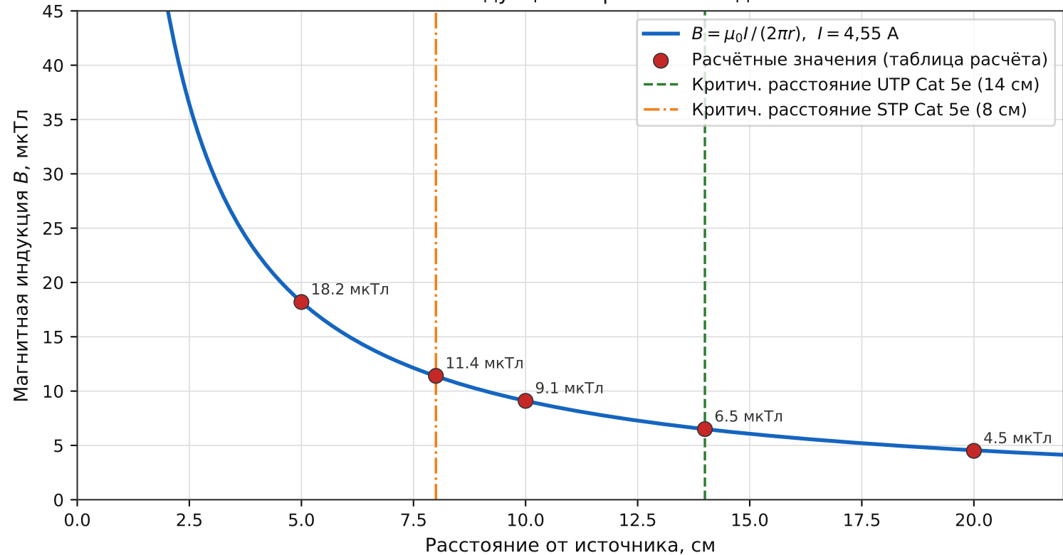
Зависимость магнитной индукции от расстояния до источника помех
