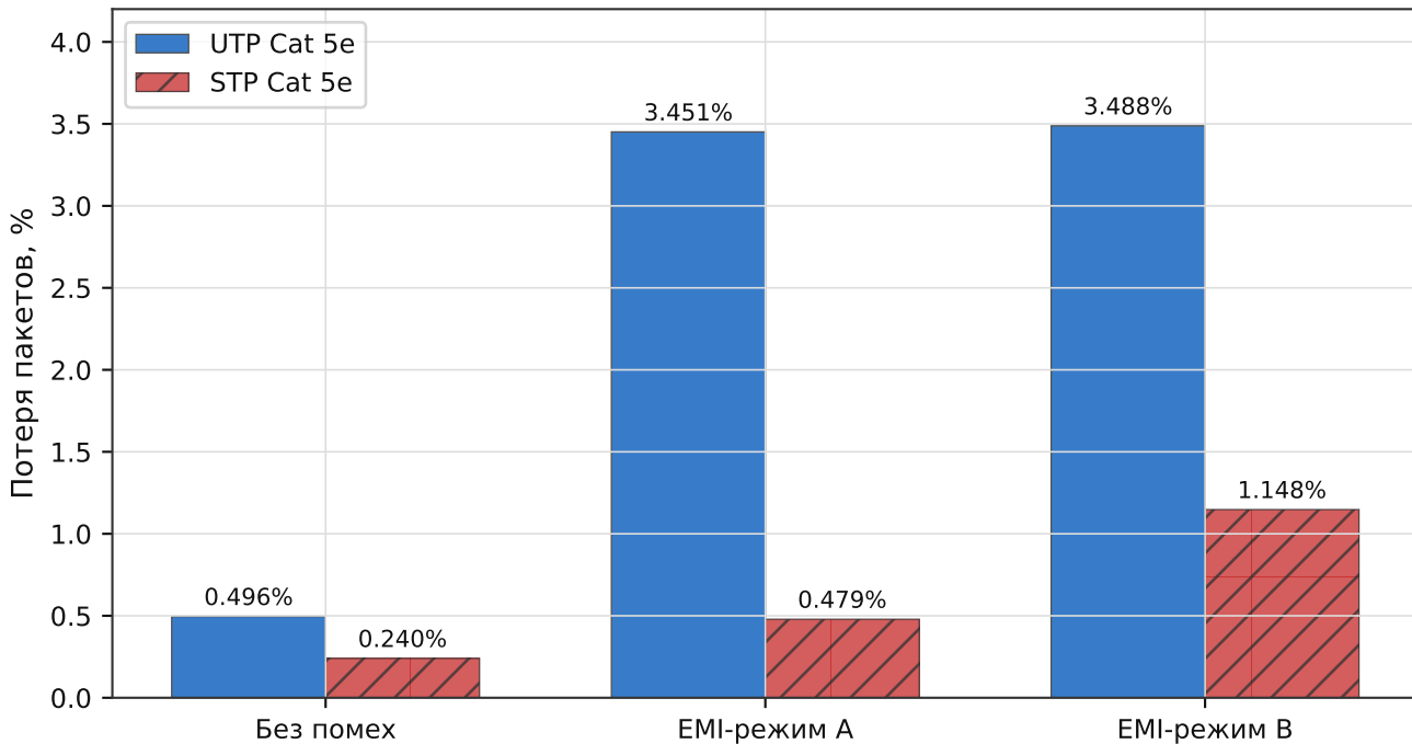
Потеря пакетов UTP и STP Cat 5e при воздействии ЭМП
