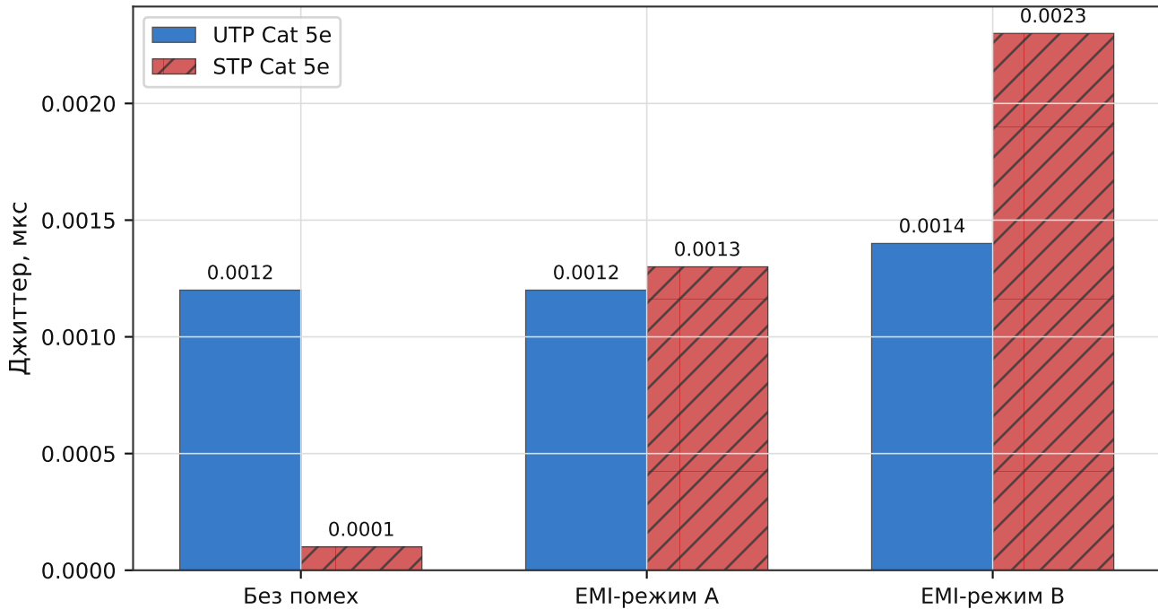
Джиттер UTP и STP Cat 5e при воздействии ЭМП
