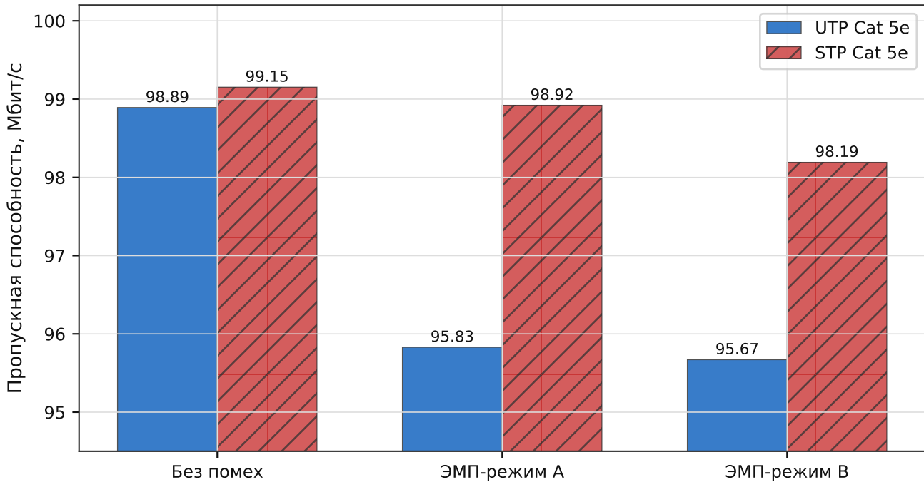
Пропускная способность UTP и STP Cat 5e при воздействии ЭМП
