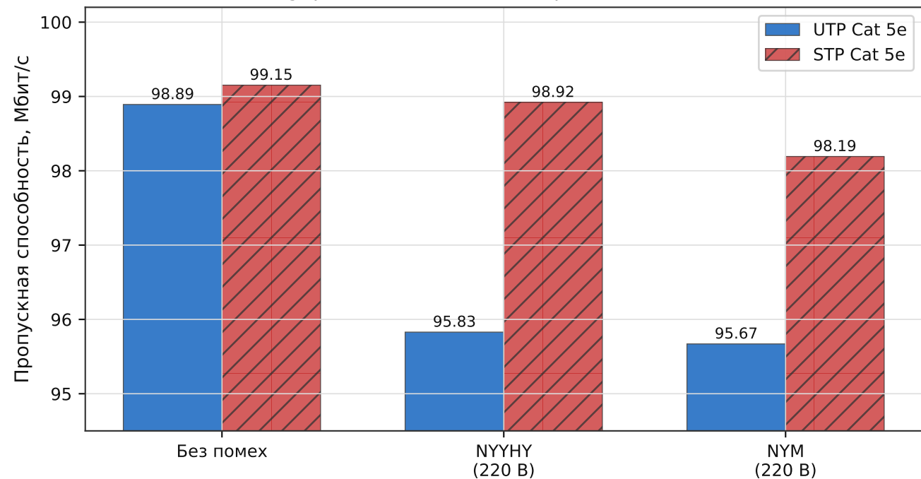
Throughput UTP и STP Cat 5e при воздействии ЭМП
