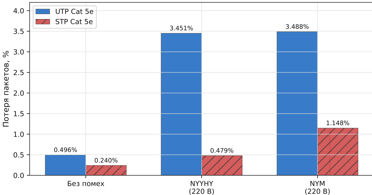
Packet Loss UTP и STP Cat 5e при воздействии ЭМП
