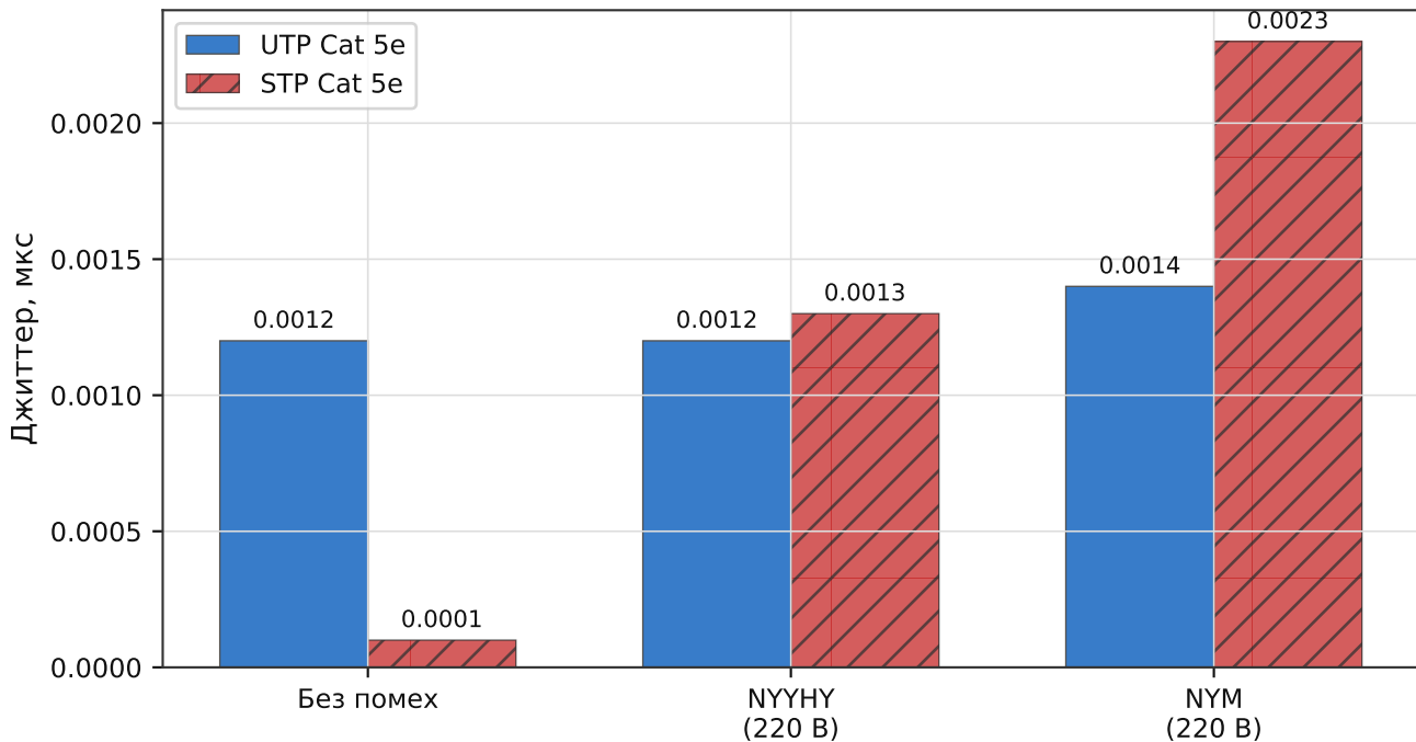
Jitter UTP и STP Cat 5e при воздействии ЭМП
