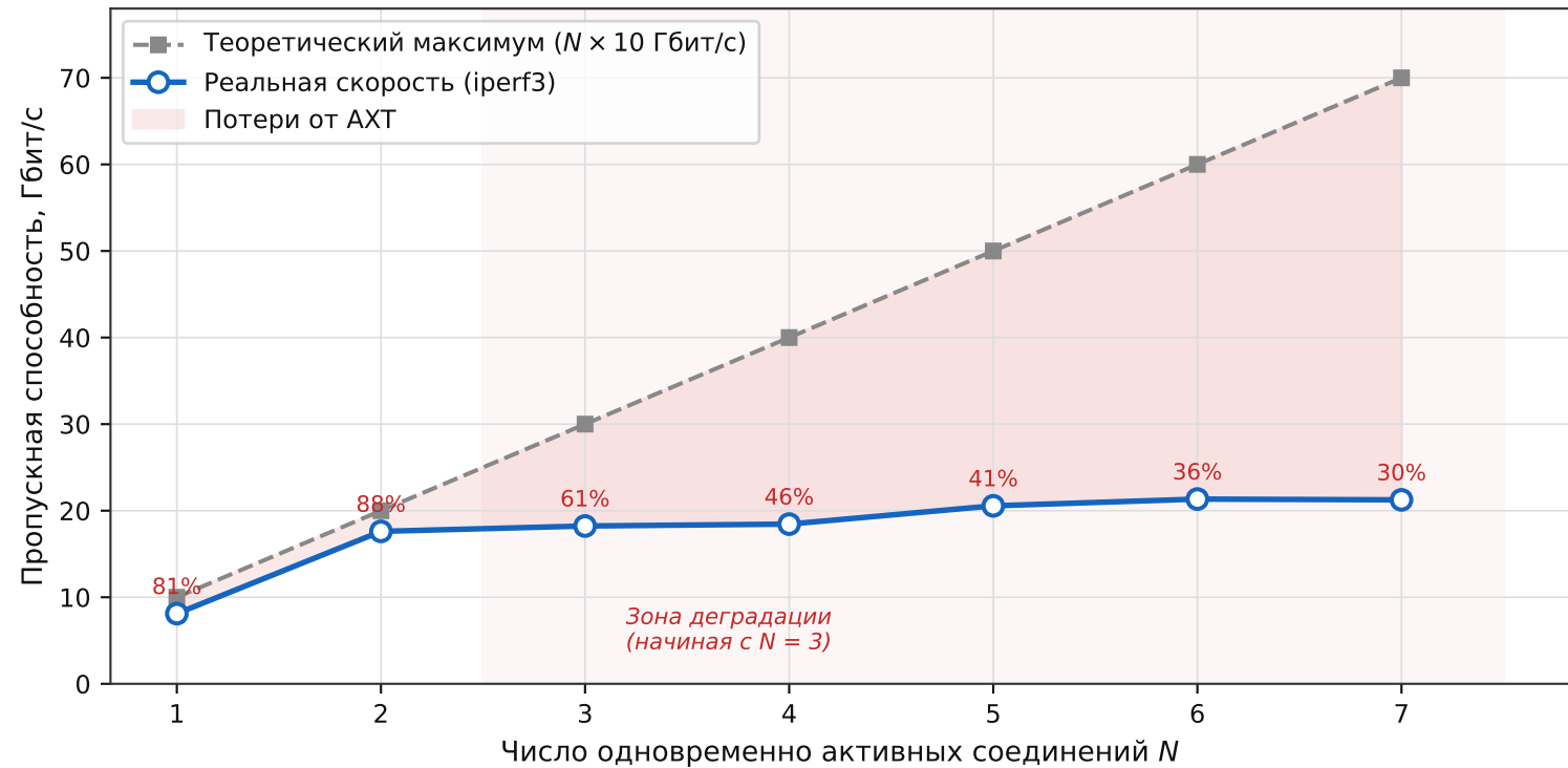
Влияние плотности кабельной укладки (AXT) на суммарную пропускную способность Cat 5e UTP, 60 м, стандарт 10GBASE-T
