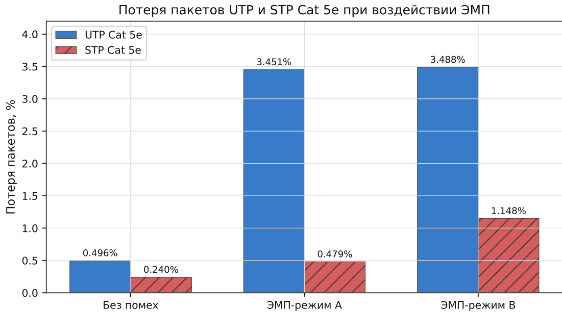
Рис. 3: Сравнение потерь пакетов UTP и STP при воздействии ЭМП
