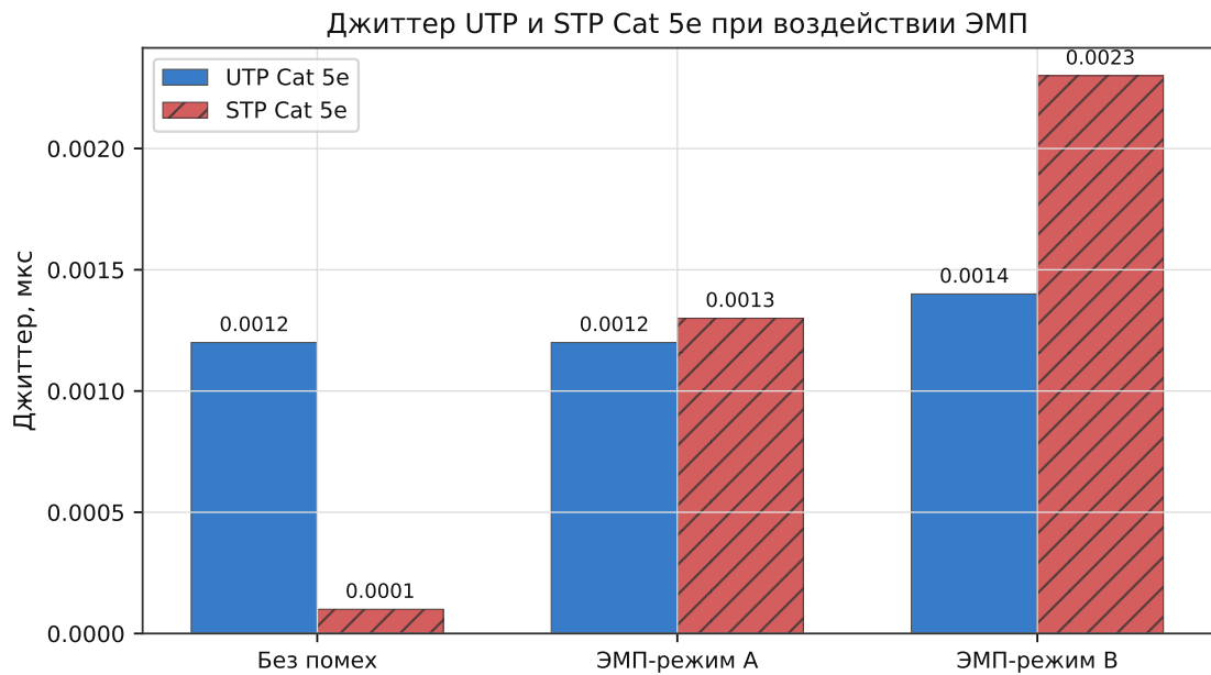
Рис. 4: Сравнение джиттера UTP и STP при воздействии ЭМП
