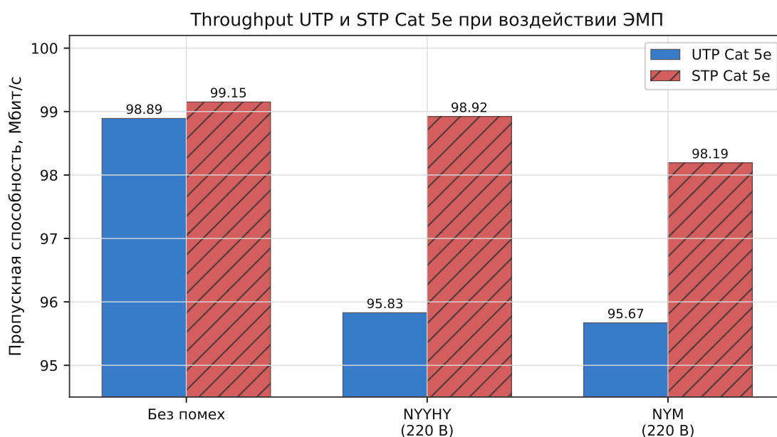
Рис. 2: Сравнение пропускной способности UTP и STP при воздействии ЭМП
