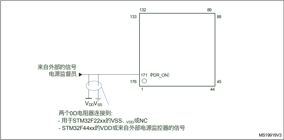
图4。用于LQFP176和BGA176封装的STM32F22xx和STM32F4xx之间的兼容板设计
