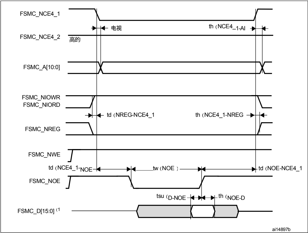
图65。用于属性存储器读取访问的PC卡/CompactFlash控制器波形
