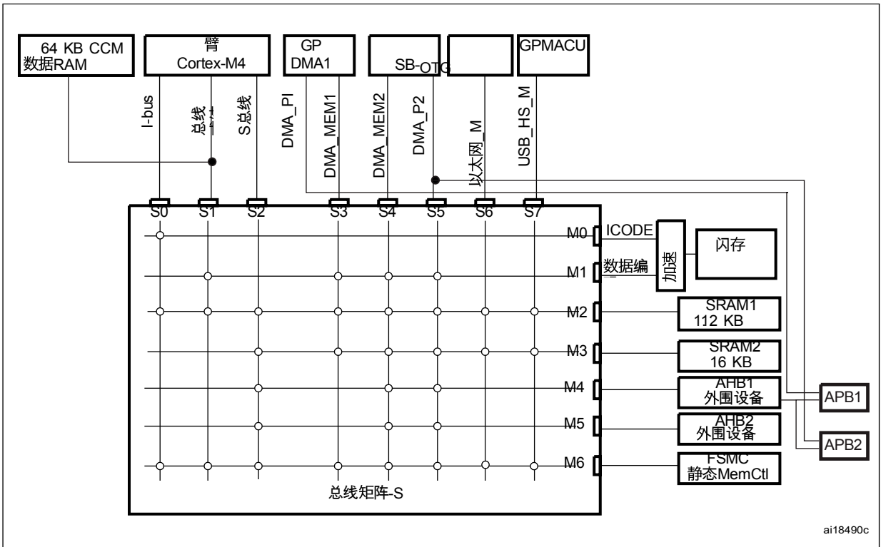
图6. 多AHB矩阵
