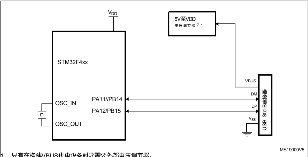
图86。USB控制器仅配置为外围设备并在全速模式下使用
