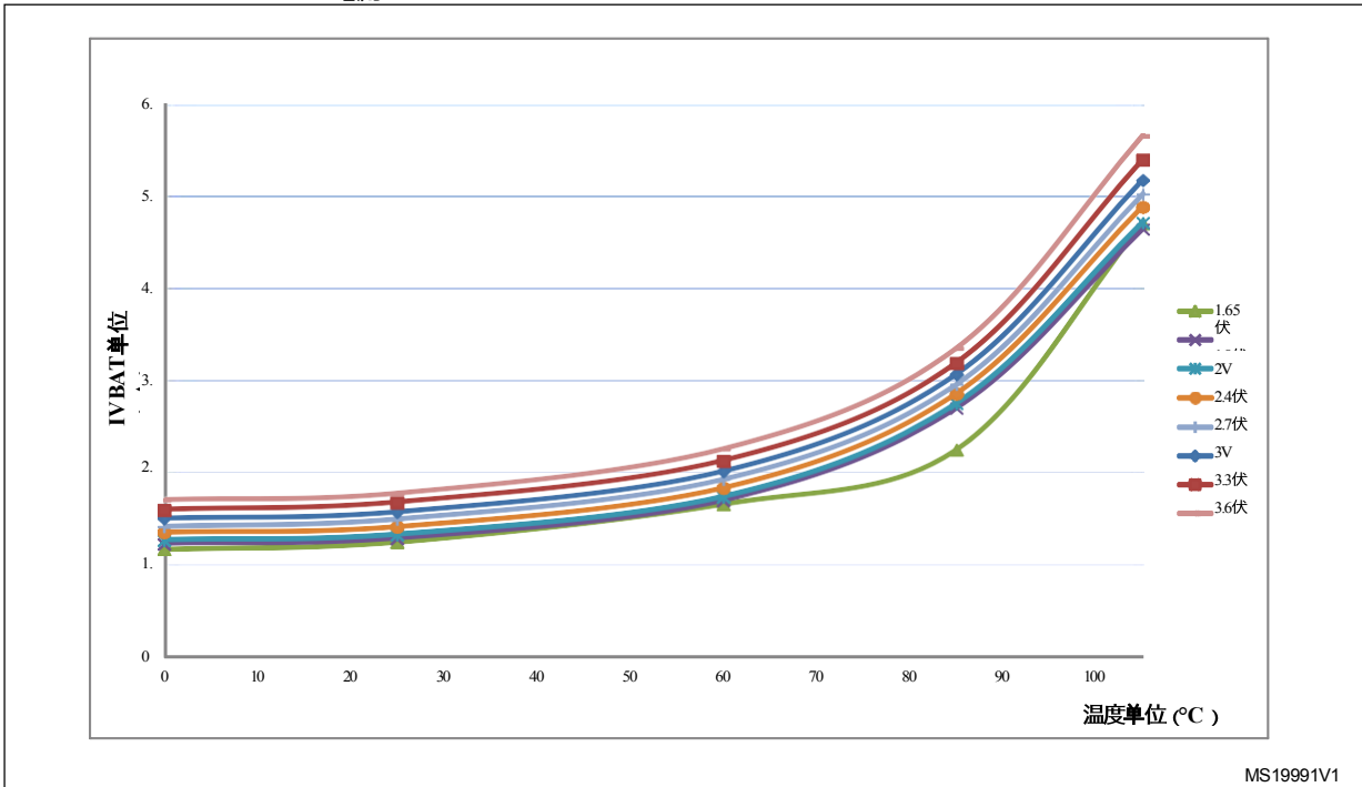
图29。典型VBAT电流消耗 (LSE和RTC开启/备份RAM开启)
