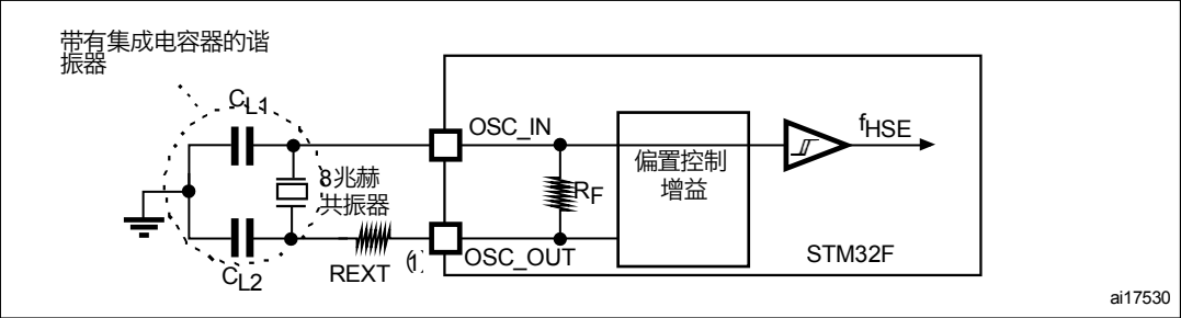
图32。8 MHz晶体的典型应用
