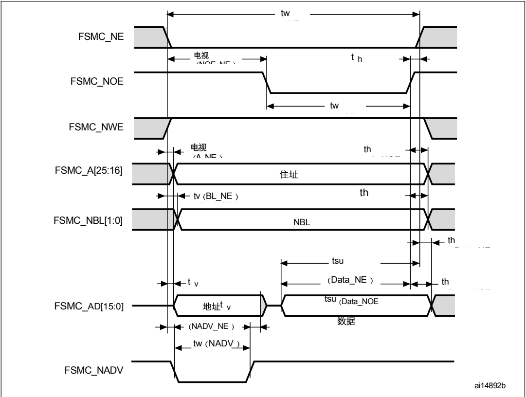
图57。异步多路复用PSRAM/NOR读取波形
