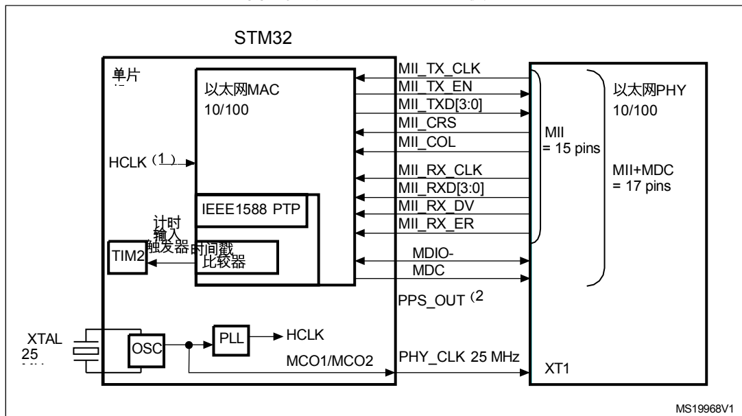
图90。使用25 MHz晶体的MII模式
