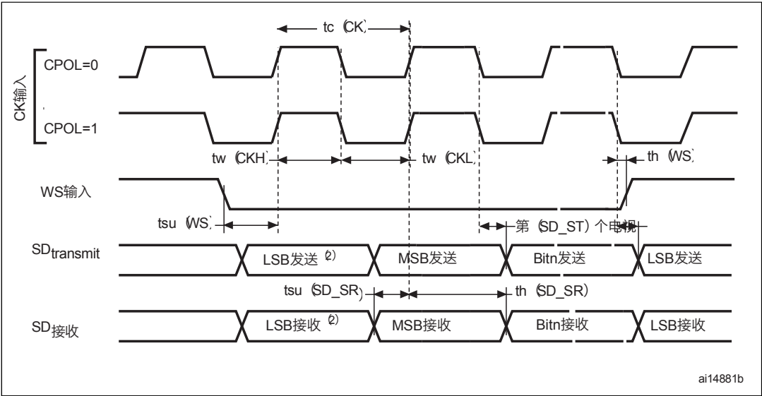
图43. I2S从时序图 (飞利浦协议)
