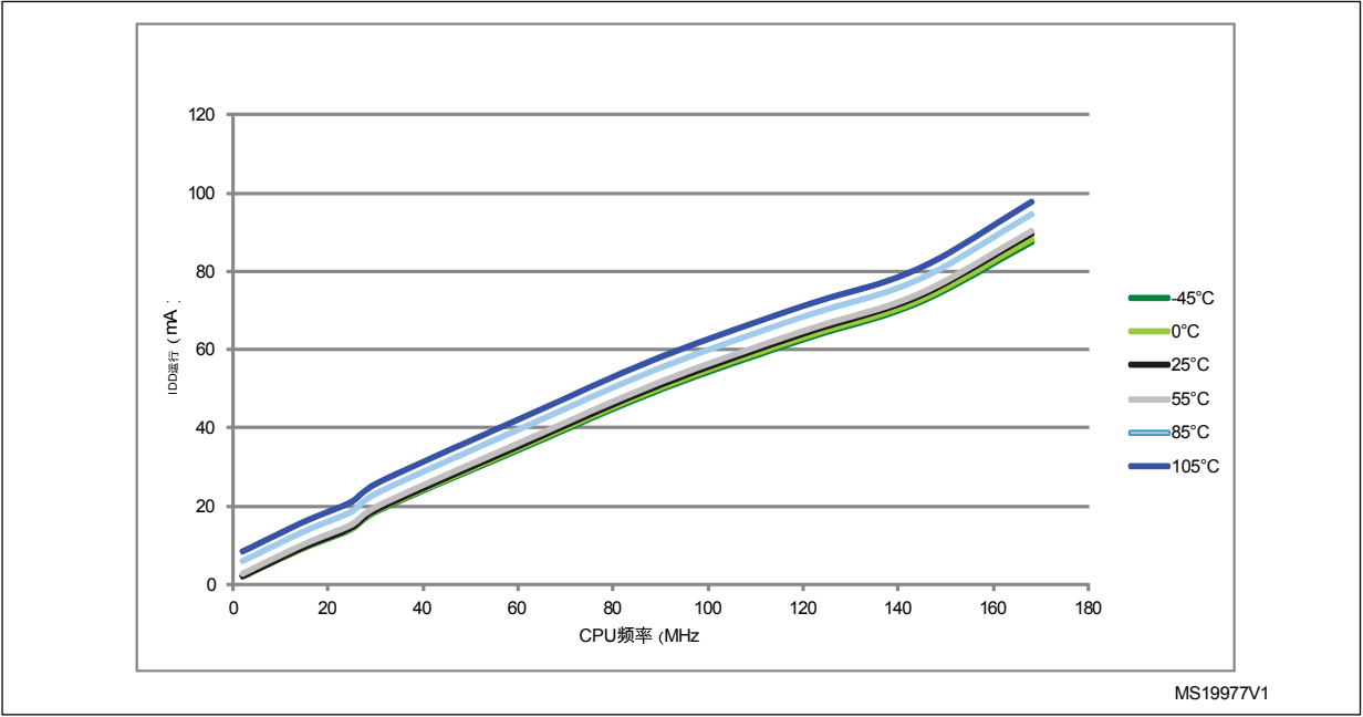
图27. 典型的电流消耗与温度、运行模式、从Flash (ART加速器关闭)或RAM运行数据处理的代码以及打开的外围设备
