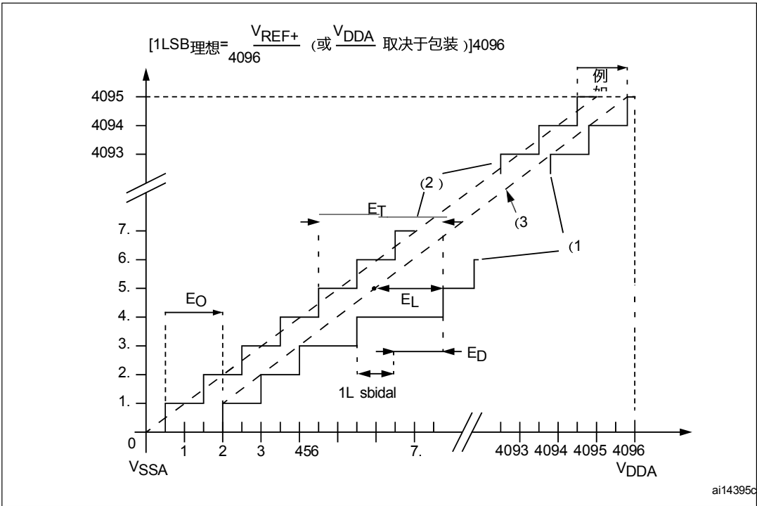
图50。ADC精度特性
