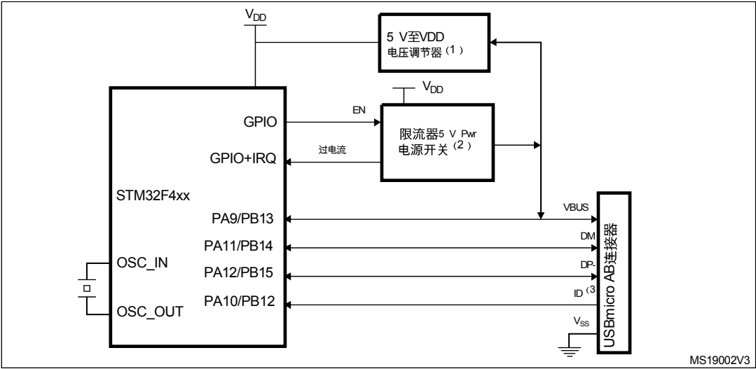
图88。USB控制器配置为双模式并在全速模式下使用
