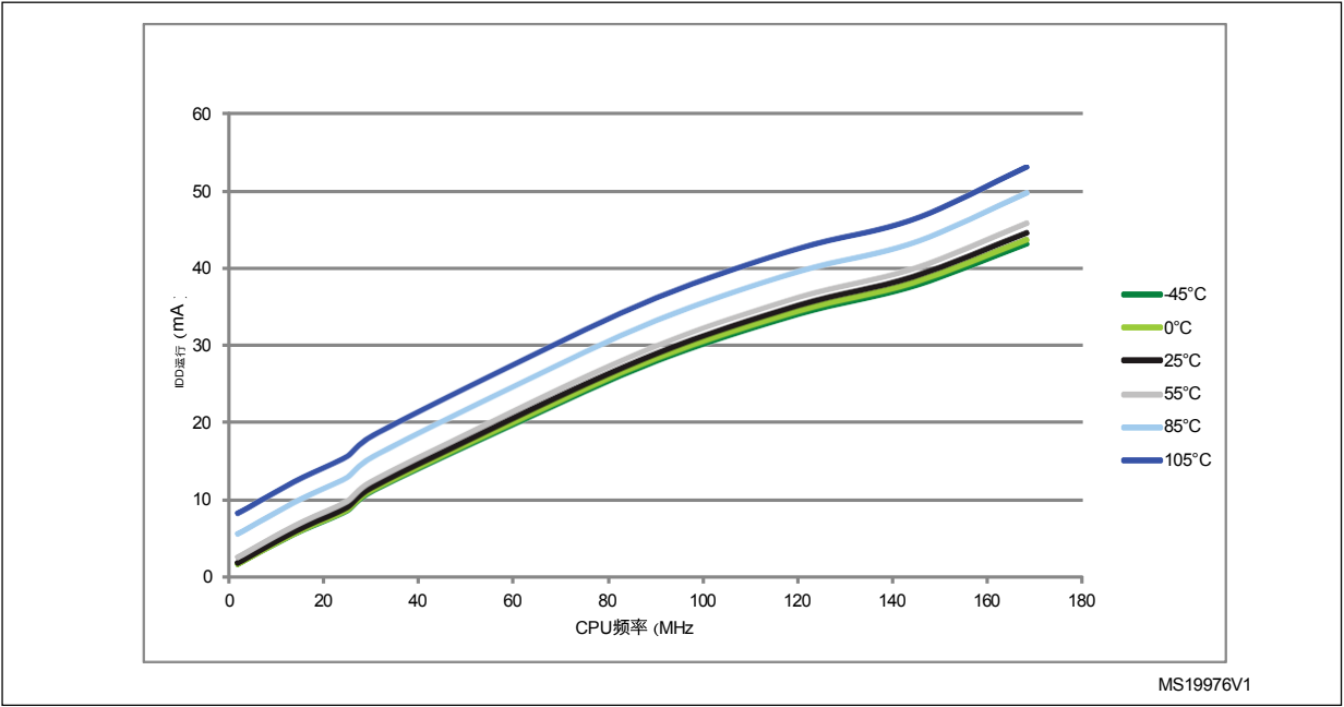
图26. 典型的电流消耗与温度、运行模式、从Flash (ART加速器关闭)或RAM运行数据处理的代码以及外围设备关闭
