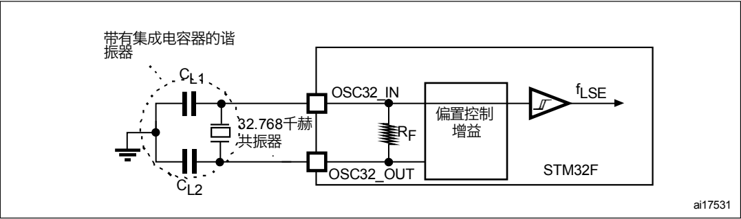
图33. 32.768 kHz晶体的典型应用
