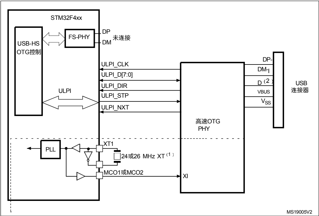
图89。USB控制器 ,配置为外设、主机或双模 ,用于高速模式
