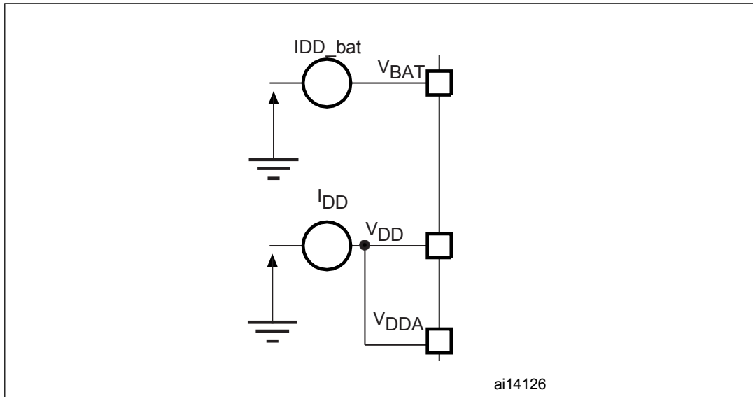
图22。电流消耗测量方案
