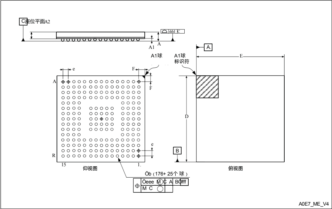
图83. UFBGA176+25-超薄细间距球栅阵列10×10×0.6mm ,封装外形
