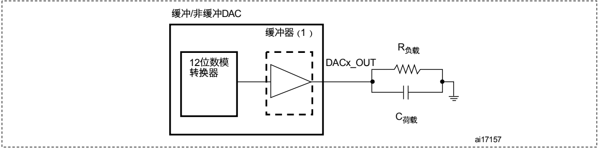
图54。12位缓冲/非缓冲DAC
