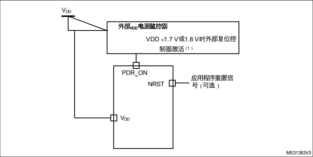
图7。内部复位关闭的电源监控器互连
