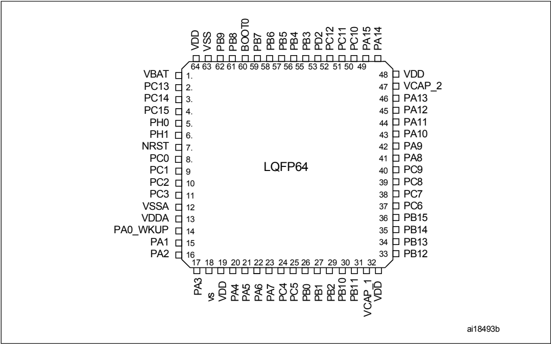
图12. STM32F40xLQFP64引脚
