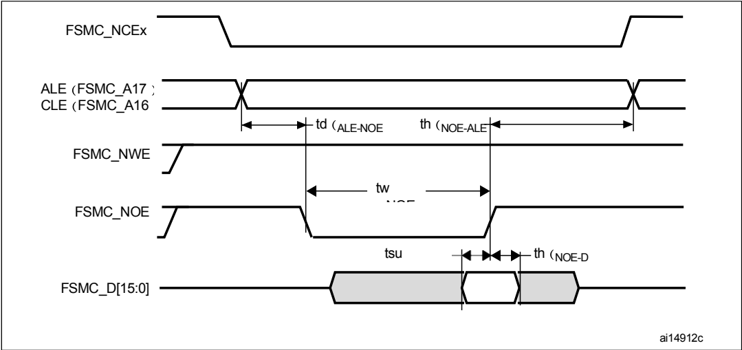
图71。用于公共存储器读取访问的NAND控制器波形
