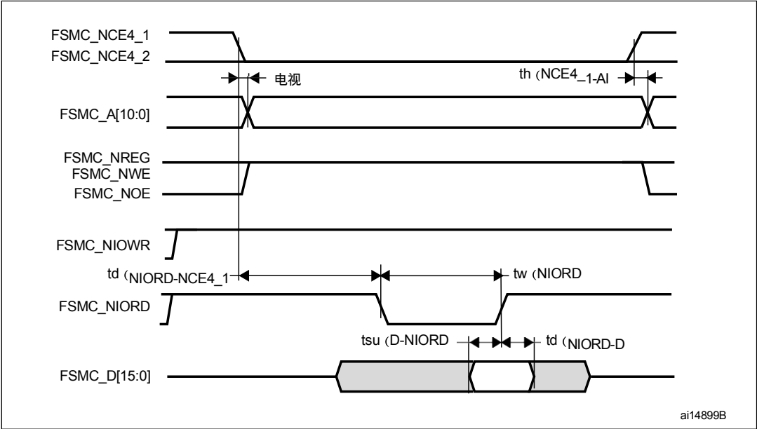
图67。用于I/O空间读取访问的PC卡/CompactFlash控制器波形
