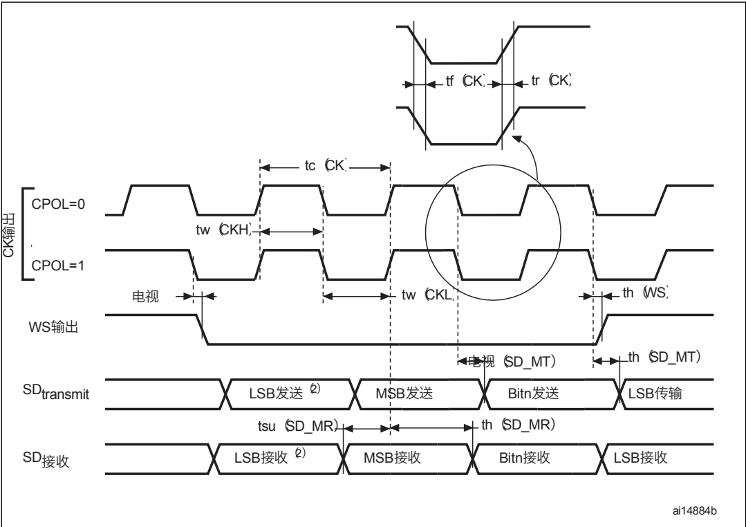
图44. I2S主时序图 (飞利浦协议) ①
