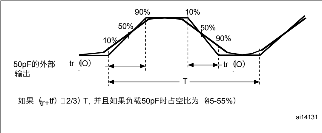
图37。I/O AC特性定义
