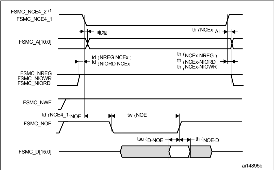
图63. 用于通用存储器读取访问的PC卡/CompactFlash控制器波形
