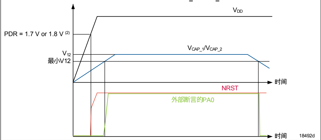
图11. 在调节器关闭模式下启动 : 快速VDD斜率 - power-down reset risen before VCAP_1/VCAP_2 stabilization
