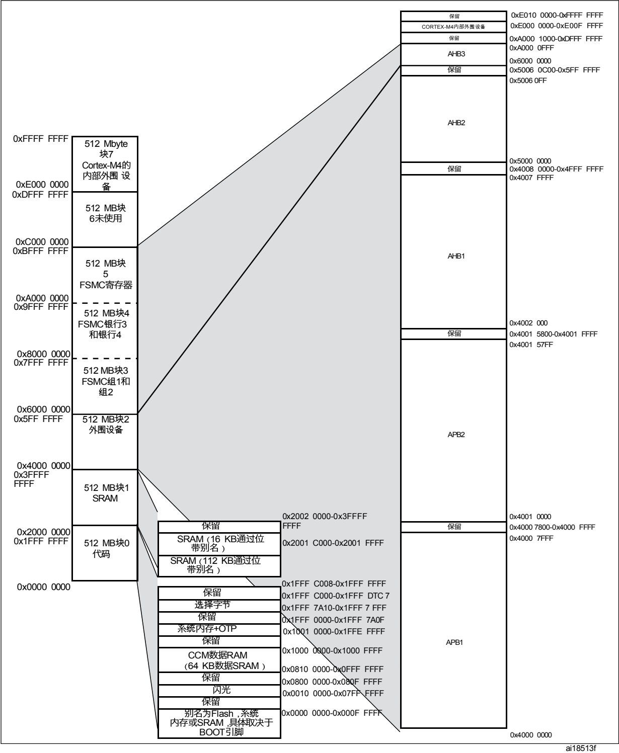
图18。STM32F40x内存映射
