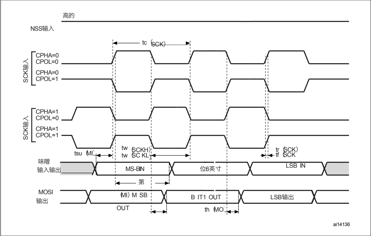
图42。SPI时序图-主模式
