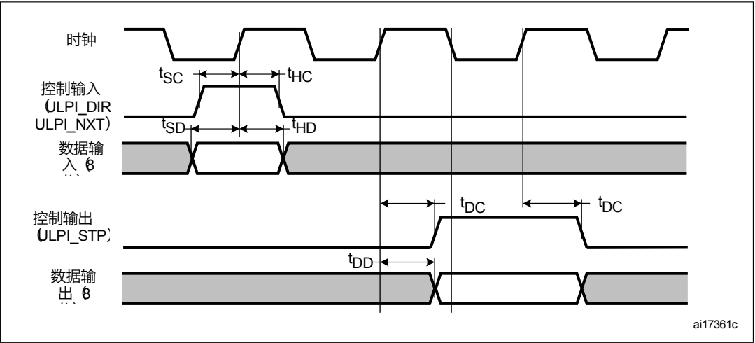
图46. ULPI时序图
