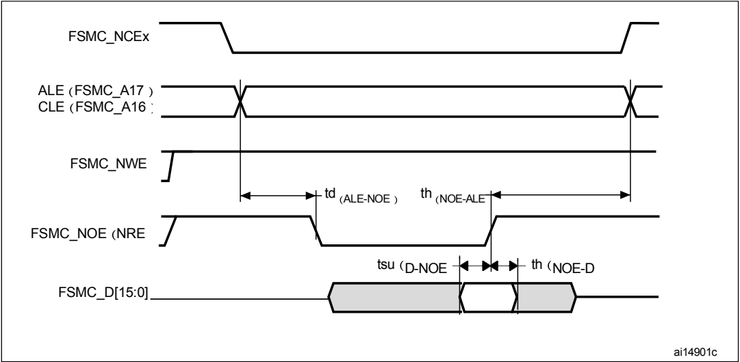
图69。用于读取访问的NAND控制器波形
