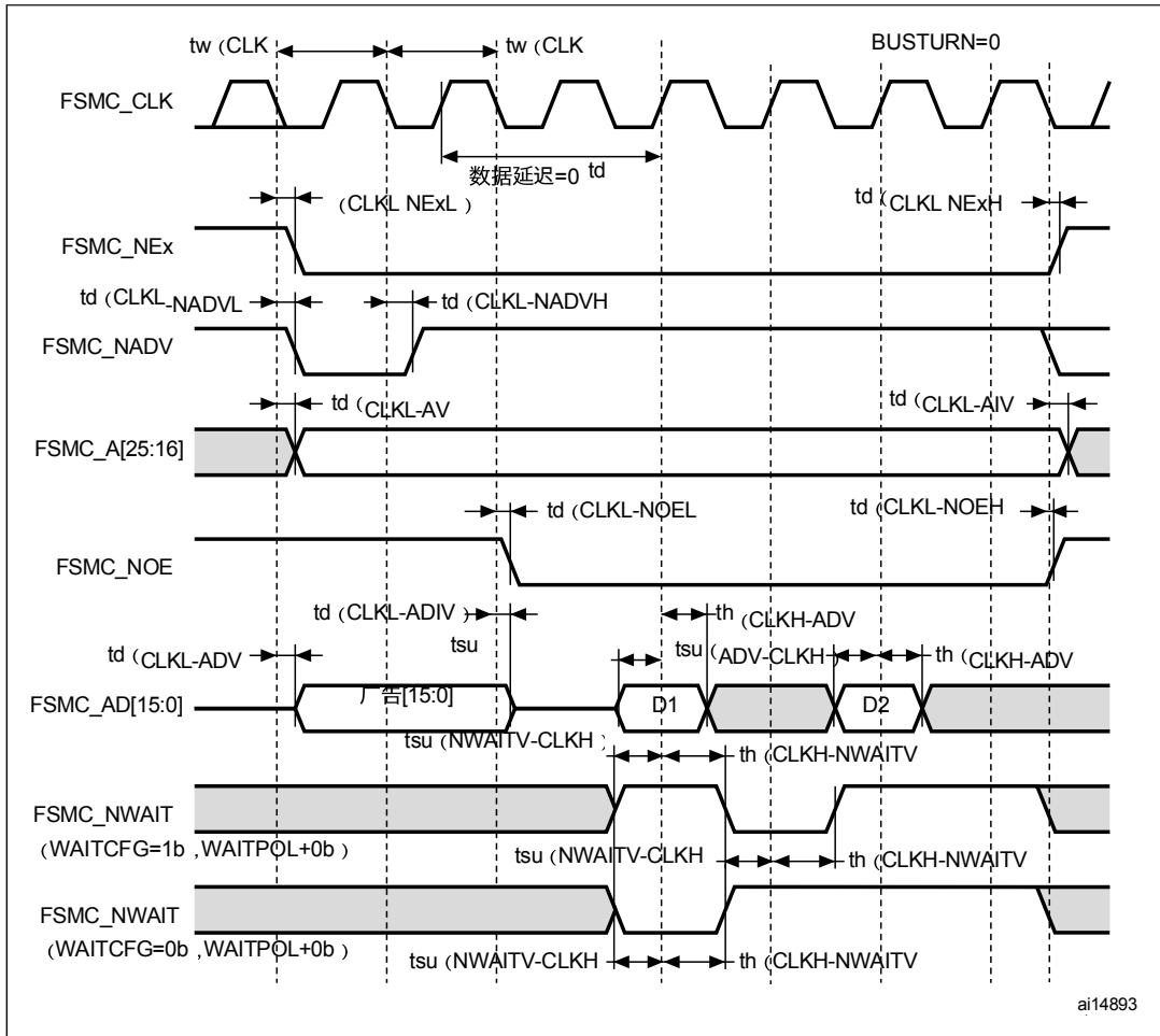
图59。同步多路复用NOR/PSRAM读取时序
