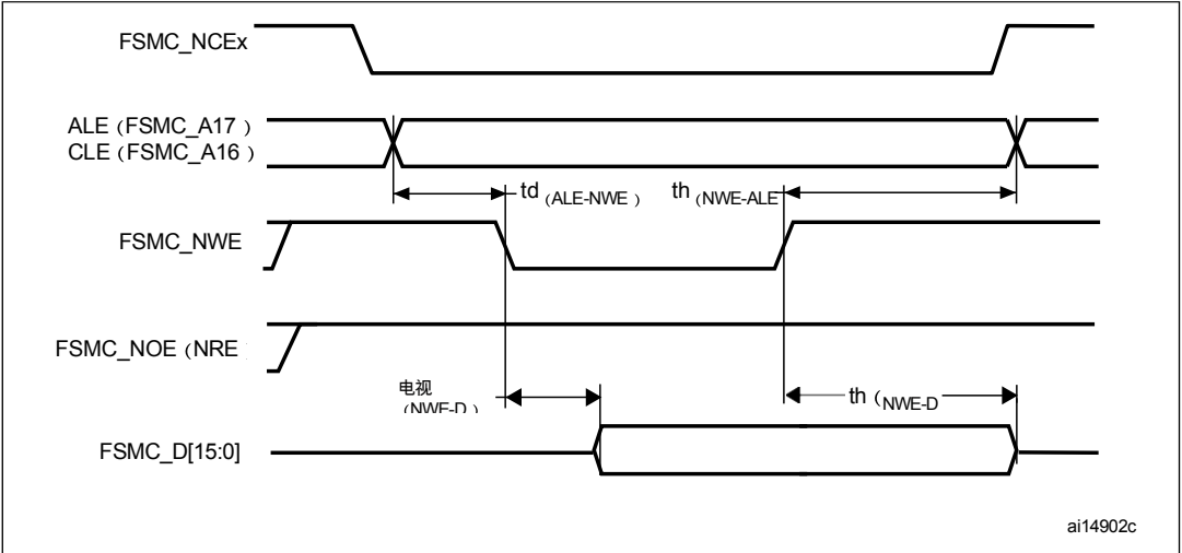
图70。用于写访问的NAND控制器波形
