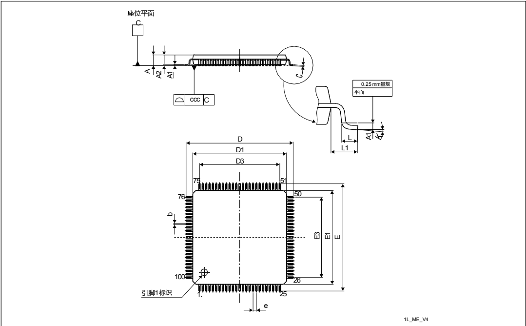
图79。LQFP100 ,14 x 14 mm 100引脚薄型四平面封装外形
