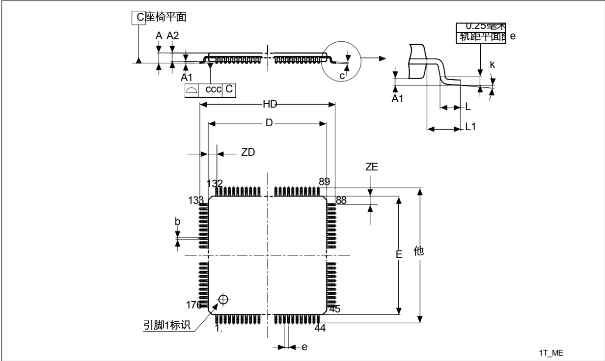
图84。LQFP176 24 x 24 mm ,176引脚薄型四平面封装外形
