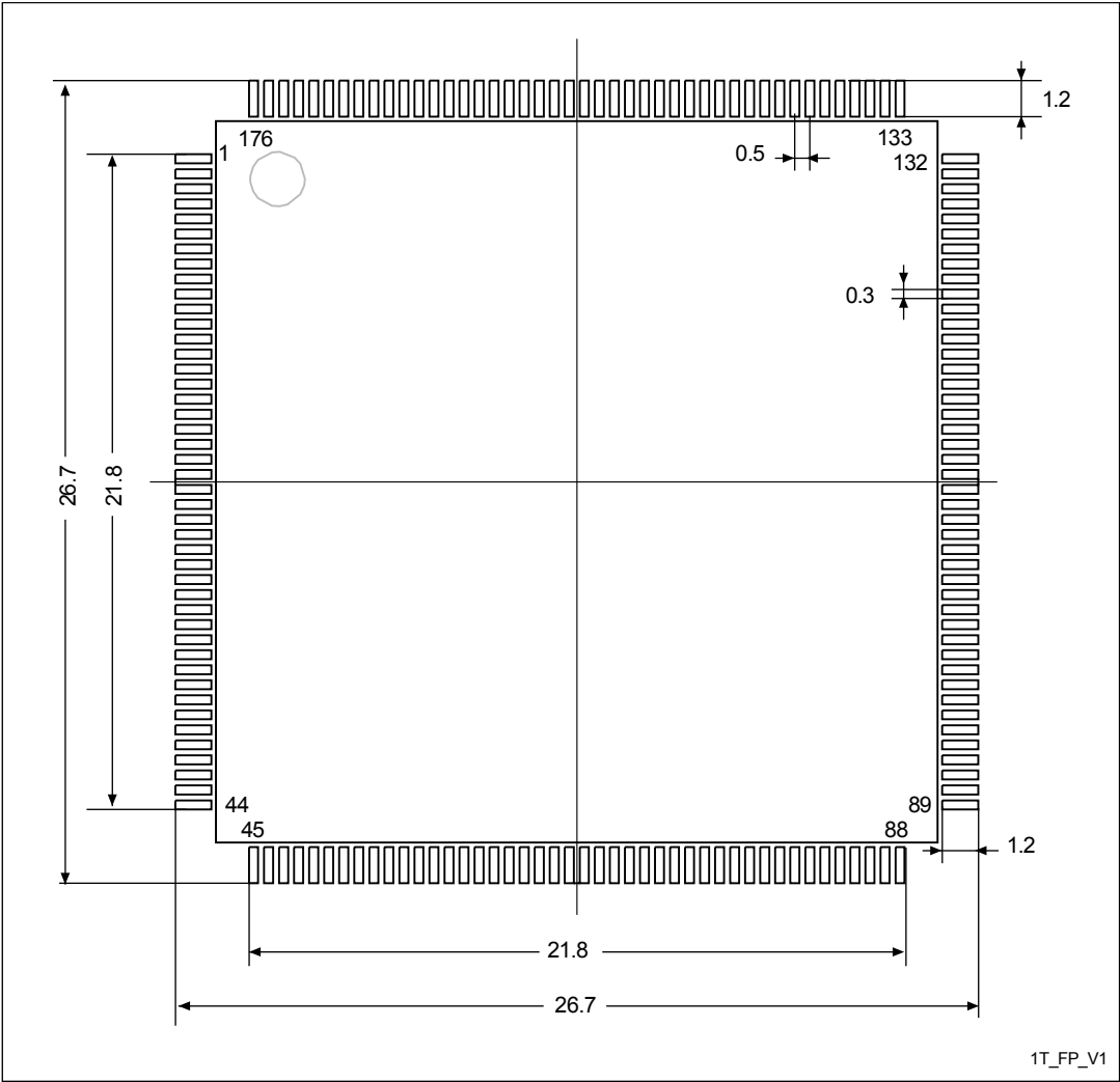
图85。LQFP176推荐的占地面积
