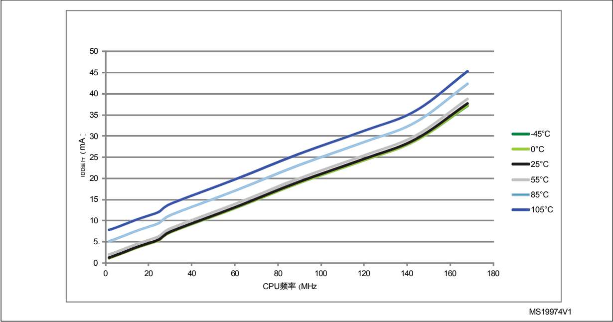
图25。典型的电流消耗与温度、运行模式、从Flash (ART加速器打开)或RAM运行数据处理的代码以及外围设备打开
