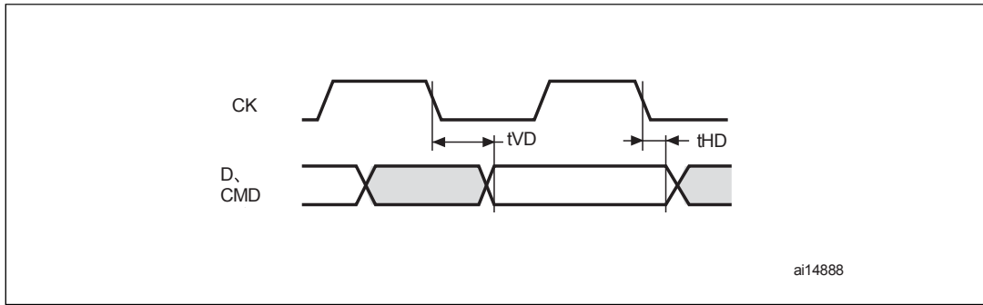
图75。SD默认模式
