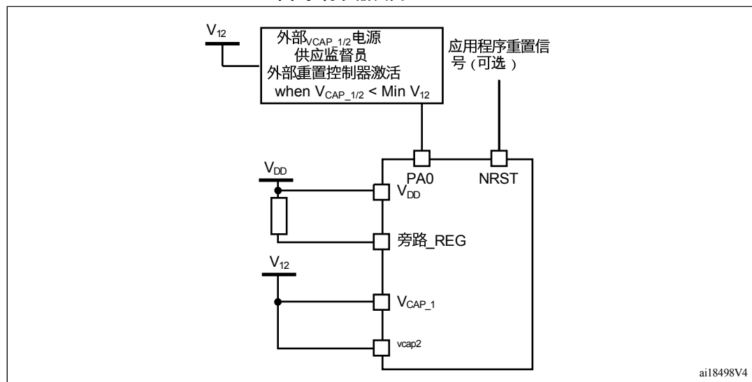
图9. 调节器关闭
