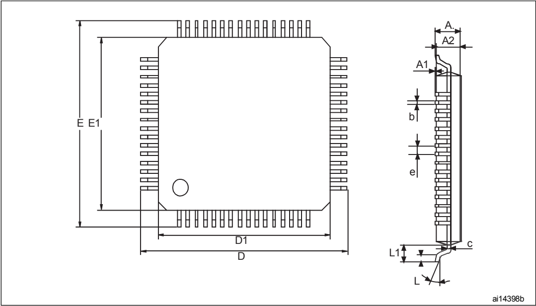
图77。LQFP64-10 x 10 mm 64引脚薄型四平面封装外形
