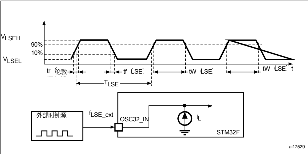
图31。低速外部时钟源交流时序图
