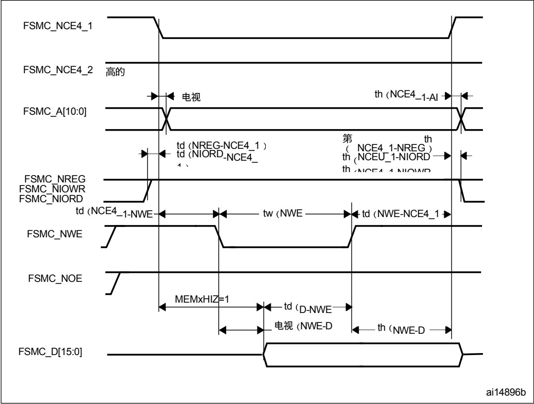
图64. 用于通用存储器写入访问的PC卡/CompactFlash控制器波形
