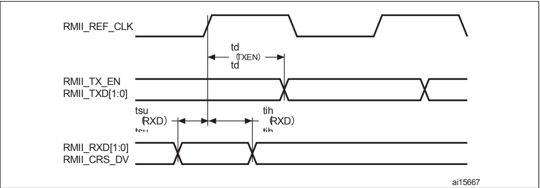
图48。以太网RMII时序图
