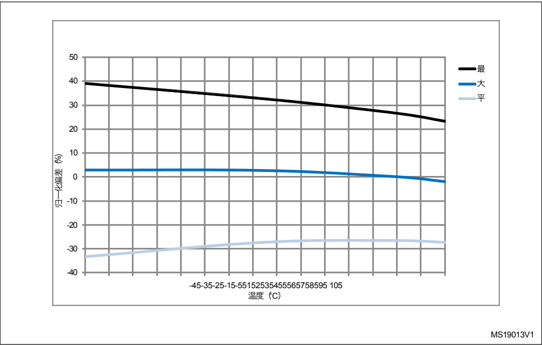
图34. ACCLSI与温度
