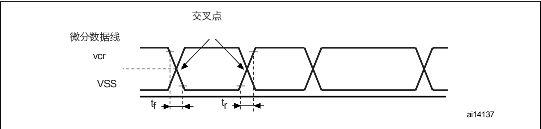
图45。USB OTG FS时序：数据信号上升和下降时间的定义
