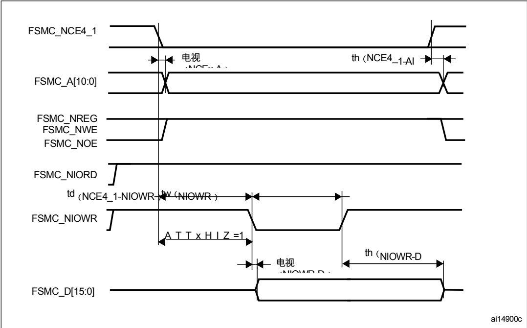
图68. 用于I/O空间写入访问的PC卡/CompactFlash控制器波形
