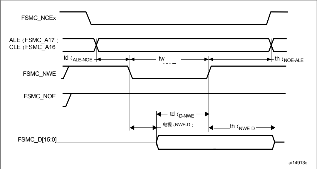
图72。用于公共存储器写入访问的NAND控制器波形
