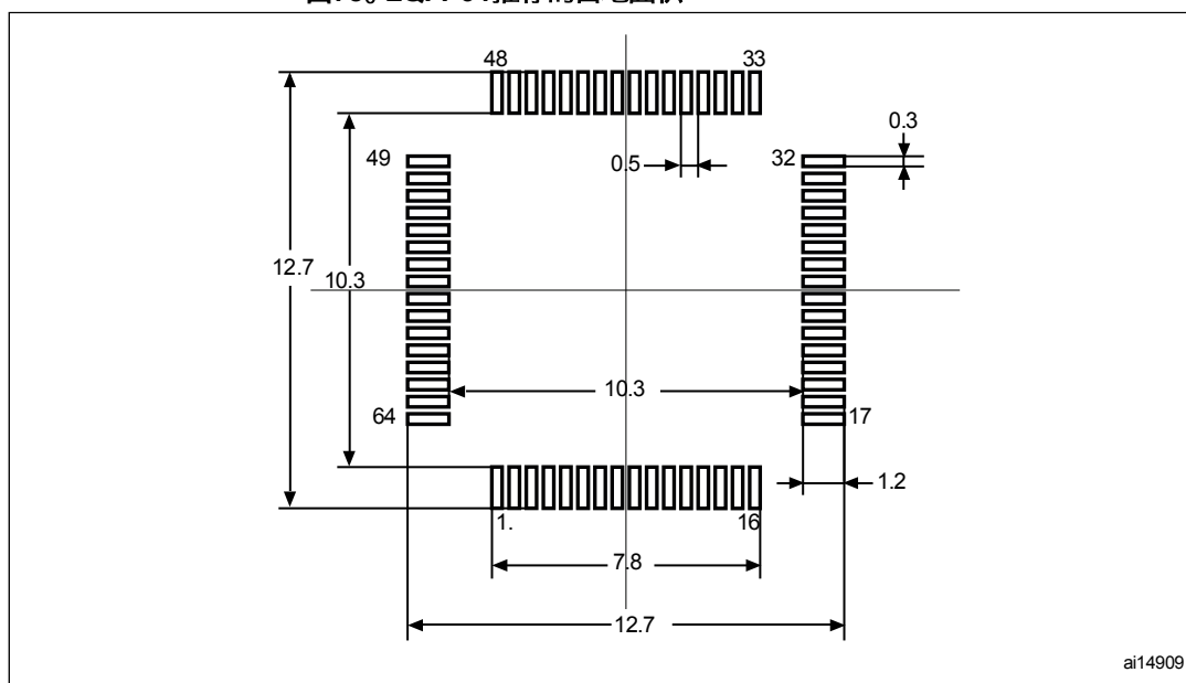
图78。LQFP64推荐的占地面积
