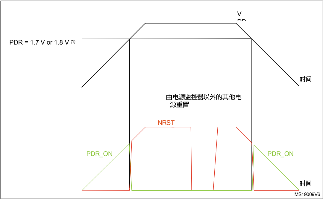
图8。内部复位关闭的PDR_ON和NRST控制
