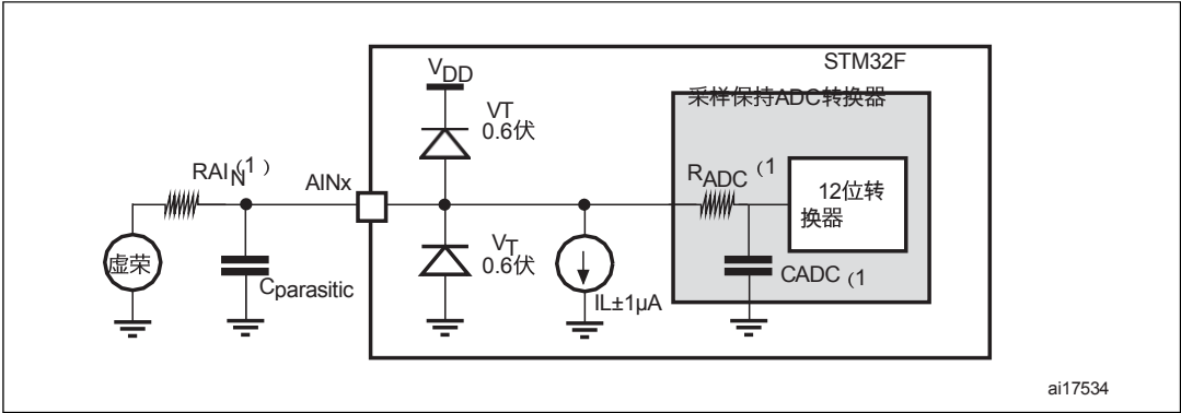
图51. 使用ADC的典型连接图
