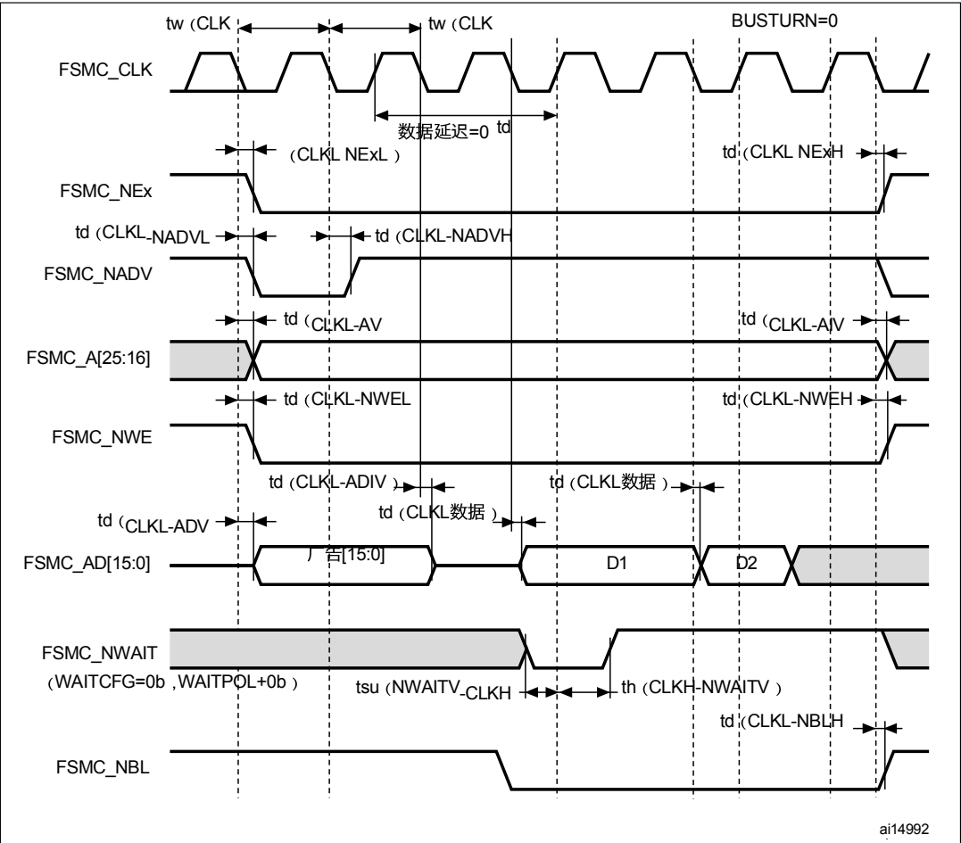
图60. 同步多路复用PSRAM写入时序
