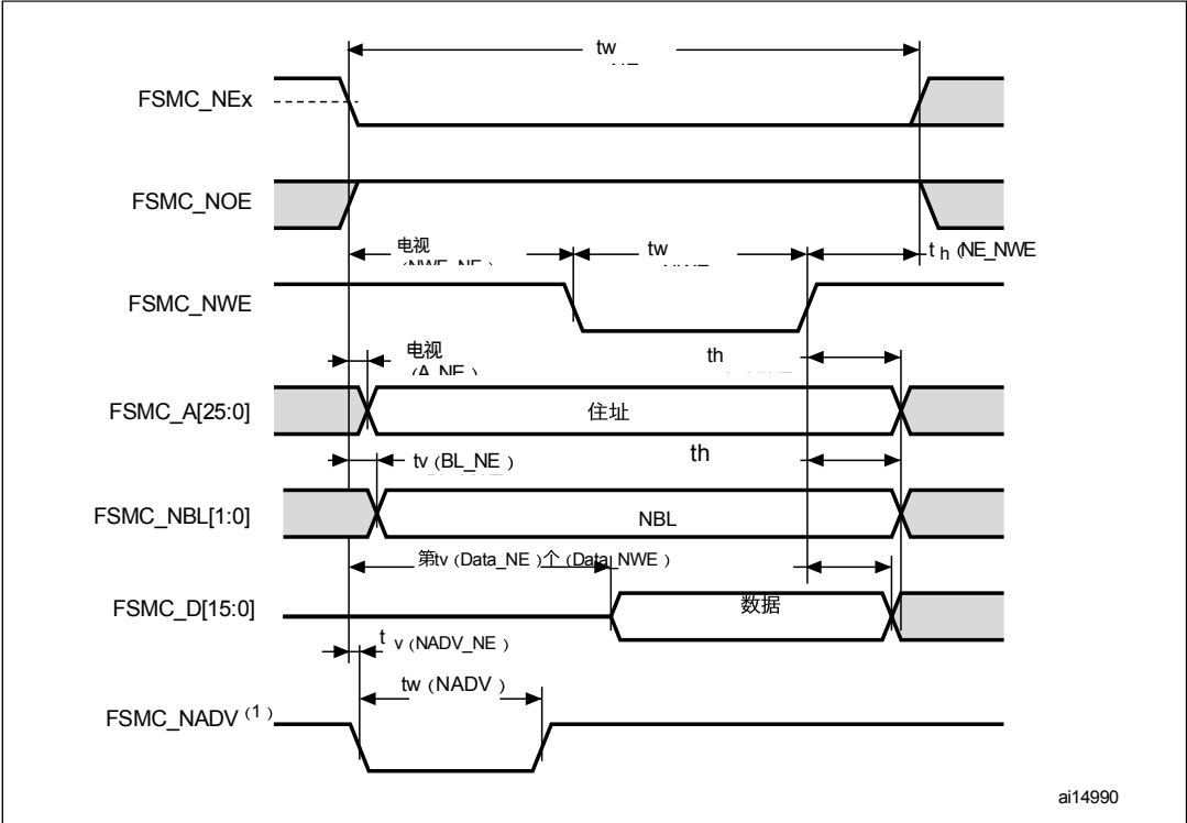
图56. 异步非多路复用SRAM/PSRAM/NOR写入波形
