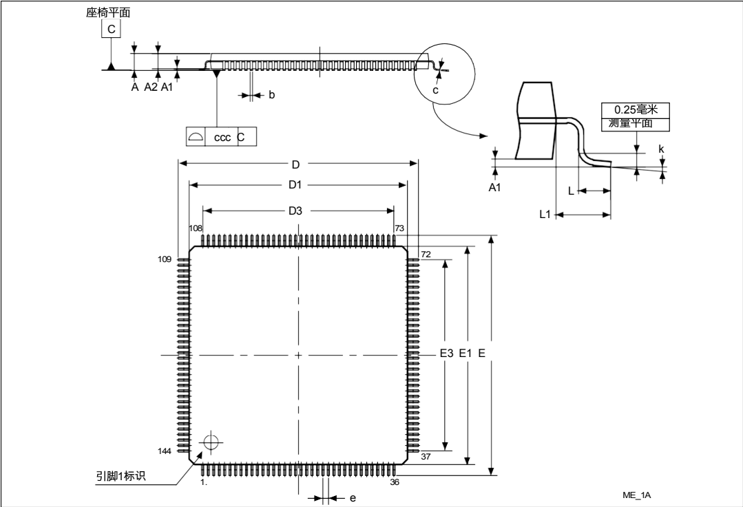
图81。LQFP144 ,20 x 20 mm ,144引脚薄型四平面封装外形
