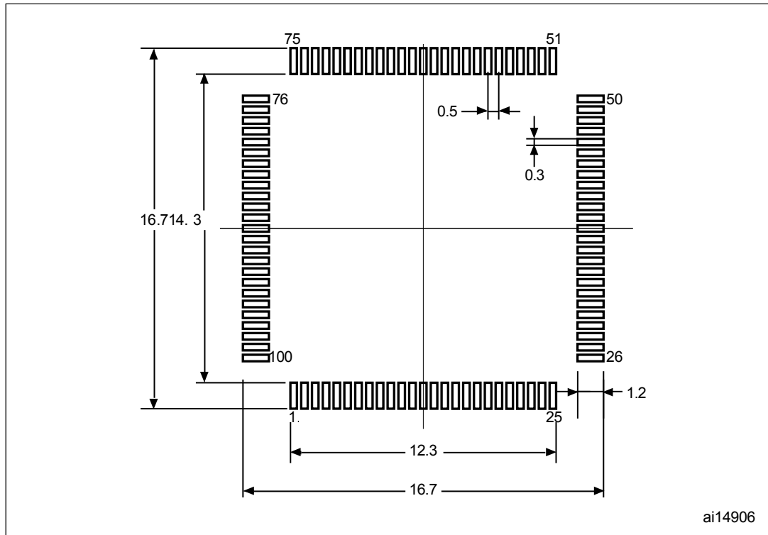
图80。LQFP100推荐占地面积
