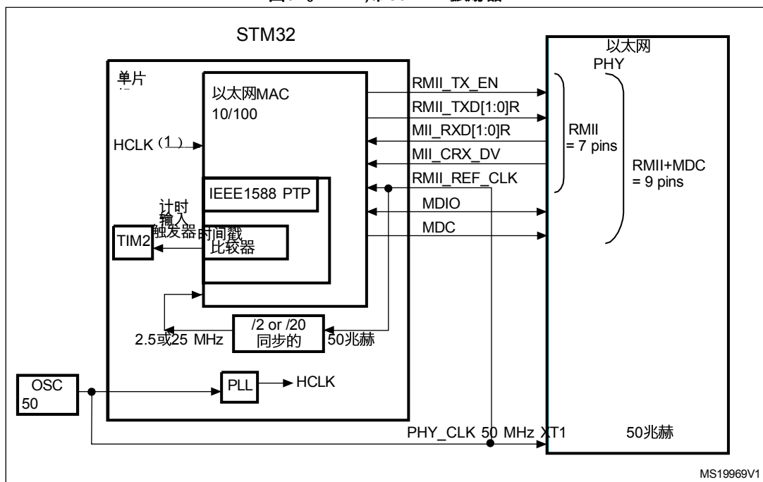
图91。RMII，带50 MHz振荡器
