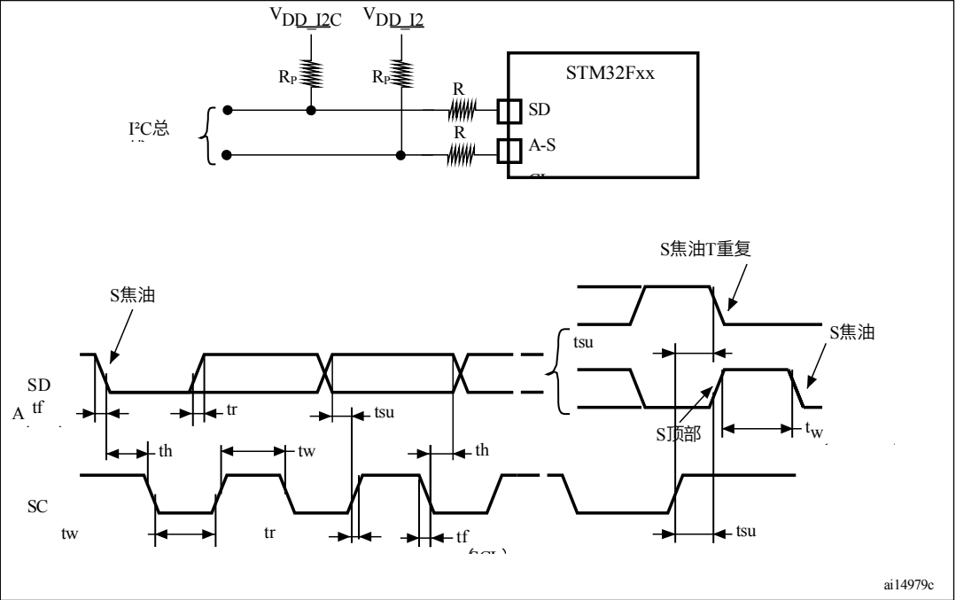
图39。I2C总线交流波形及测量电路
