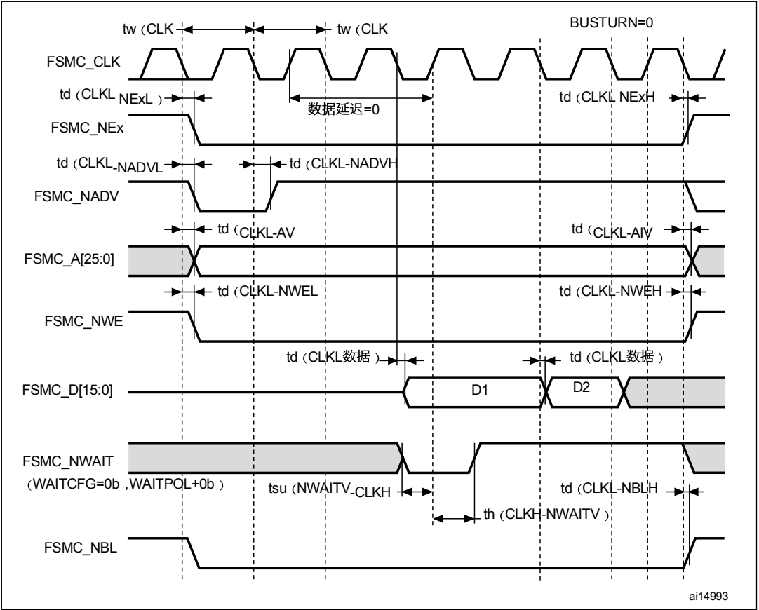
图62。同步非多路复用PSRAM写入时序
