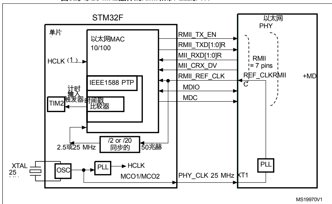
图92。带25 MHz晶体的RMII和带PLL的PHY
