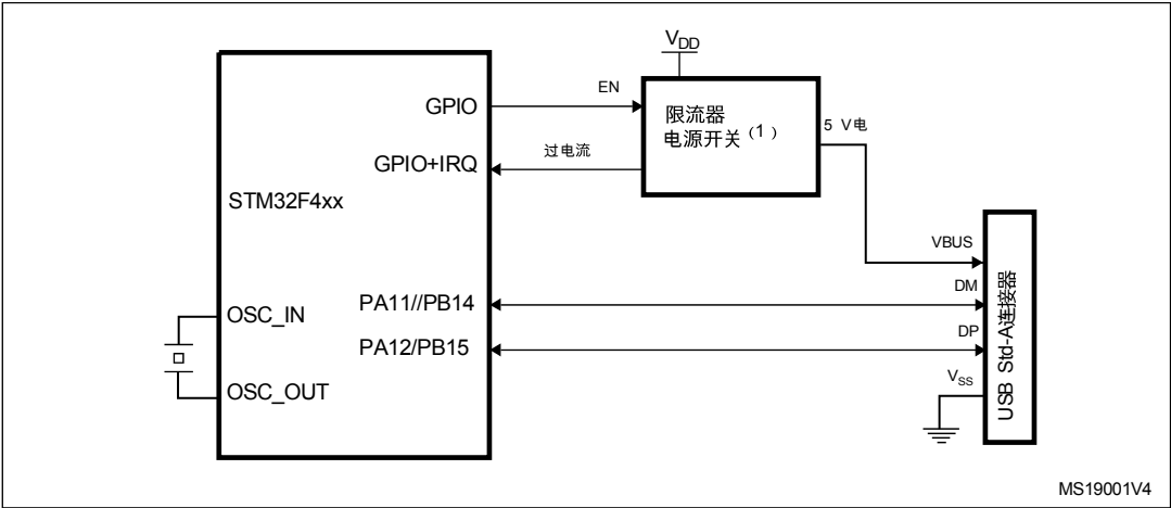
图87。USB控制器仅配置为主机并在全速模式下使用
