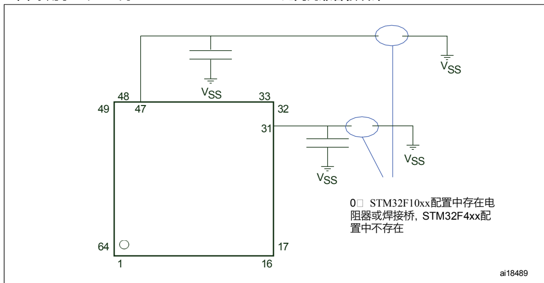
图1. 用于LQFP64的STM32F10xx/STM32F4xx之间的兼容板设计
