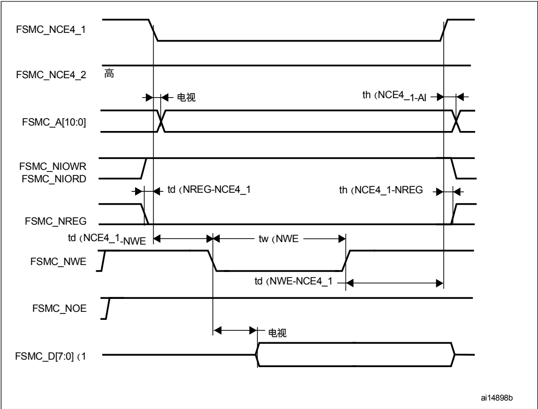
图66。用于属性存储器写入访问的PC卡/CompactFlash控制器波形
