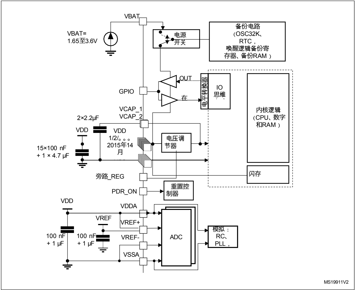
图21。供电方案
