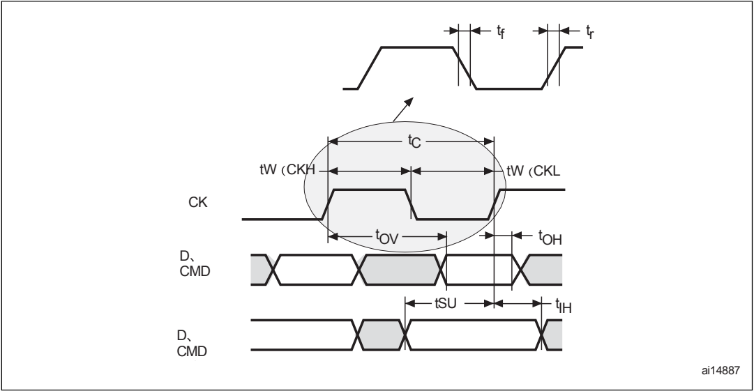
图74。SDIO高速模式
