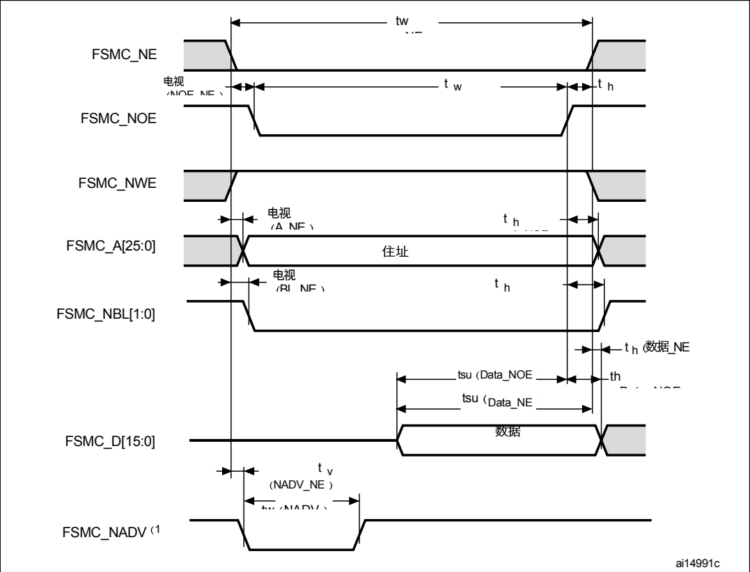
图55. 异步非多路复用SRAM/PSRAM/NOR读取波形
