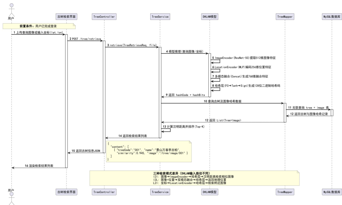
图 4.10 古树名木多模态检索时序图
