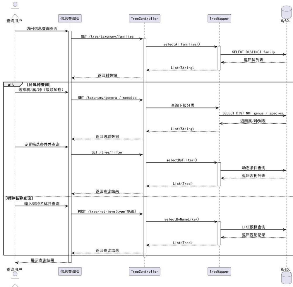
图 4.9 古树名木信息查询时序图
