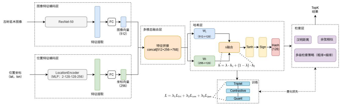
图 3.1 DHLM 模型架构
