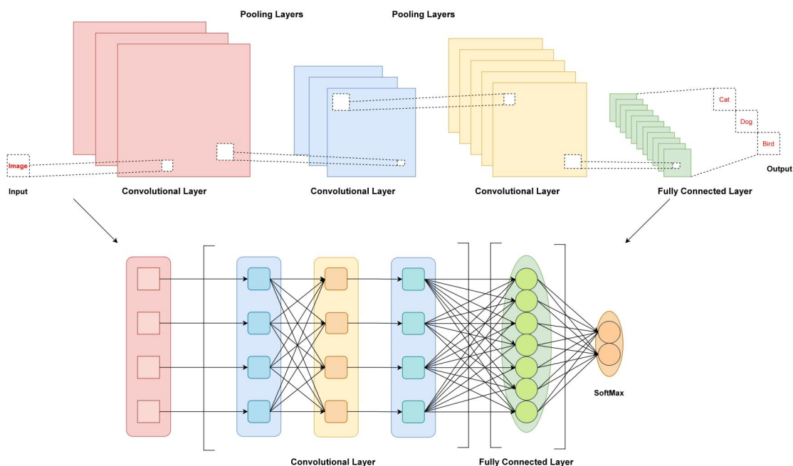
图 2.3 卷积神经网络结构
