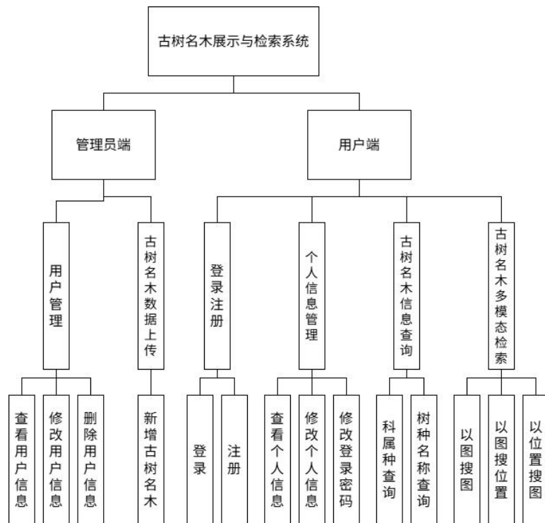
图 4.3 系统功能模块设计
