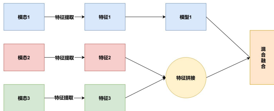
图 2.12 混合融合
