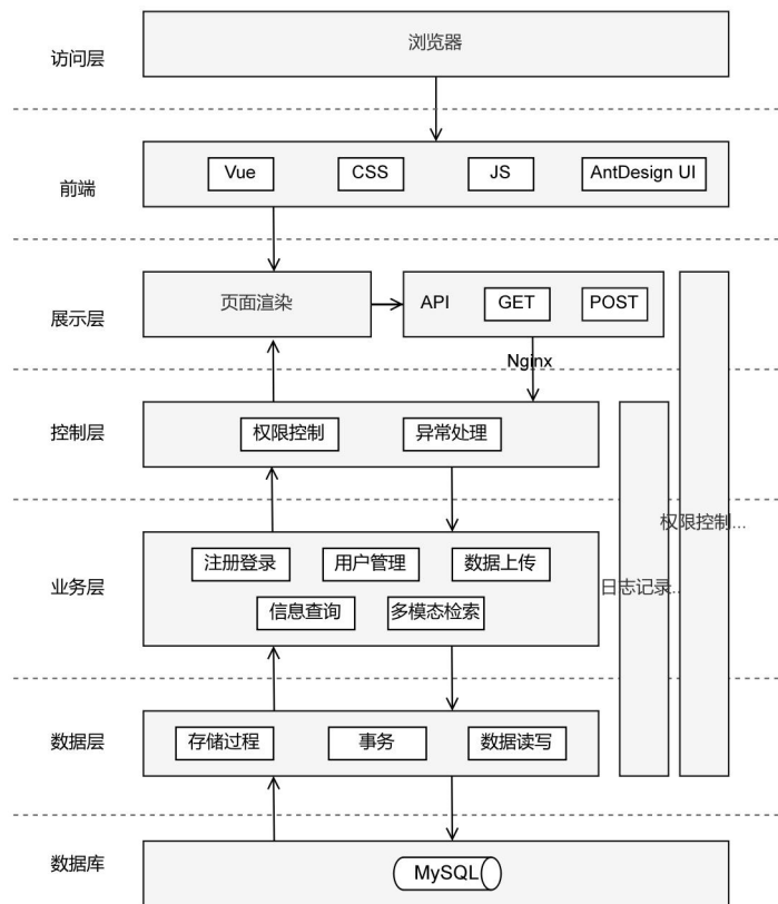
图 4.2 系统架构图
