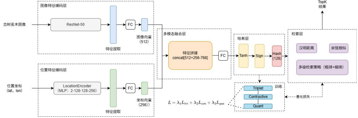
图 3.1 DHLM 模型架构
