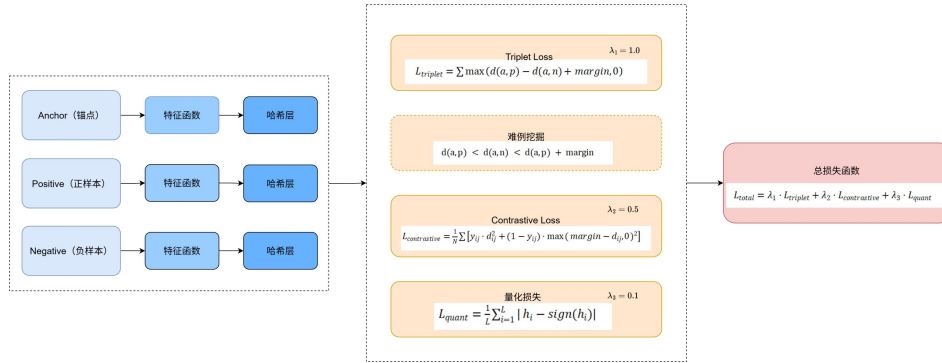
图 3.2 损失函数计算过程
