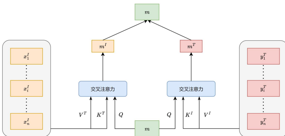
图 2.14 多步交叉注意力融合
