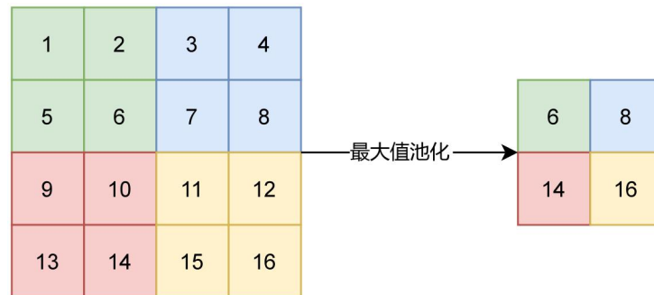
图 2.2 最大值池化
