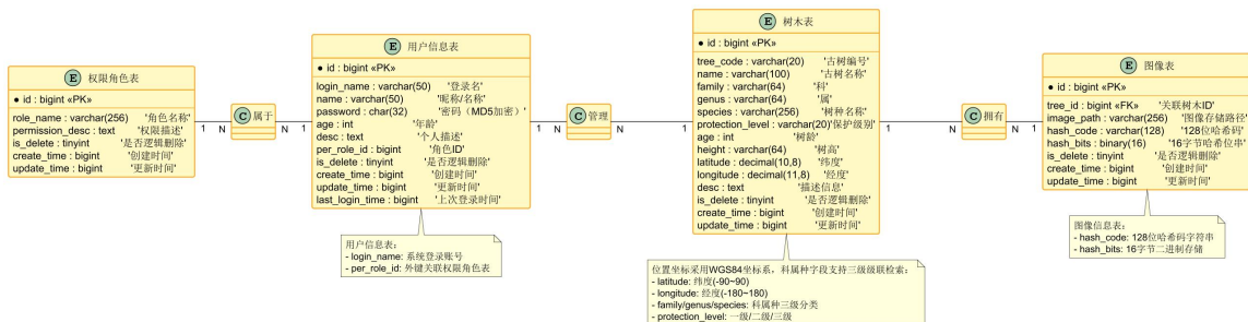
图 4.4 系统 ER 图
