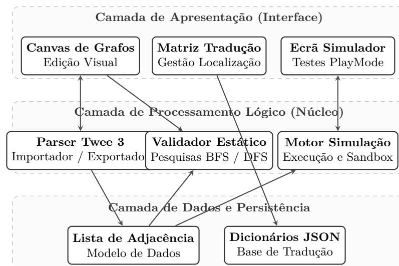
Figura 3.1: Diagrama de blocos detalhado da arquitetura conceptual e fluxo de dados.
