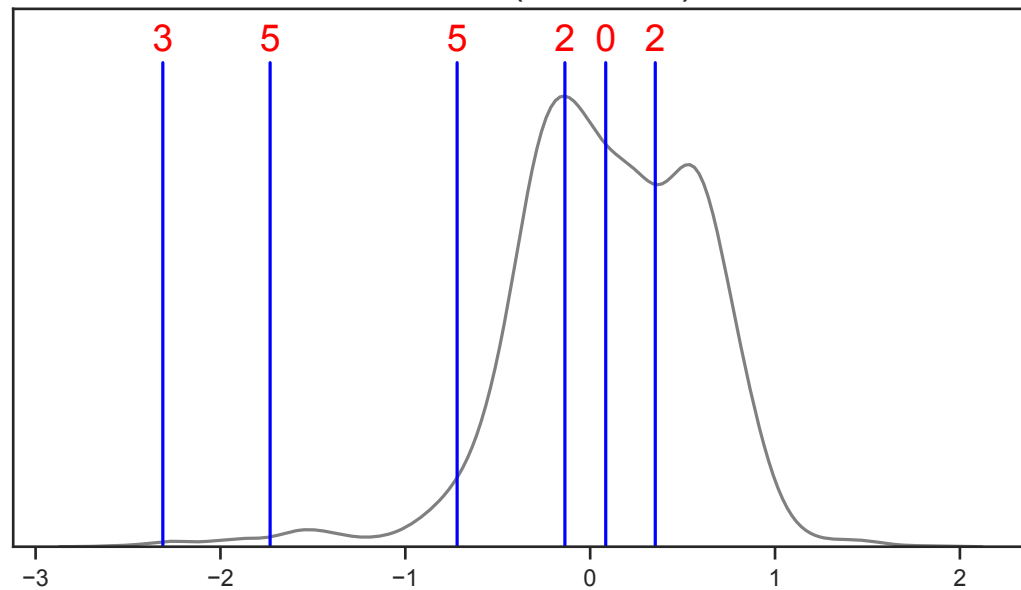
NPFFR1 (Dolcetto)
