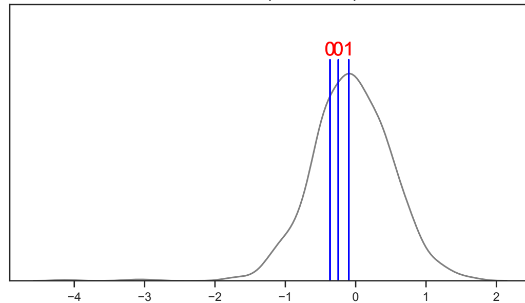
NPFFR1 (Katsano)
