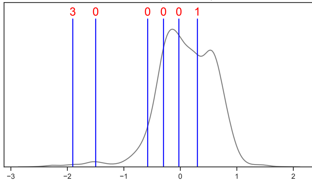
NPFFR1 (Dolcetto)
