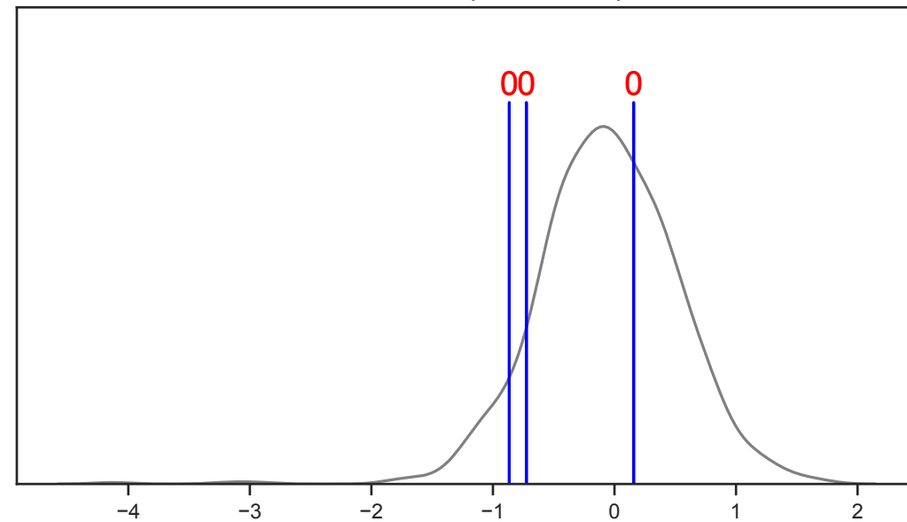
NPFFR1 (Katsano)
