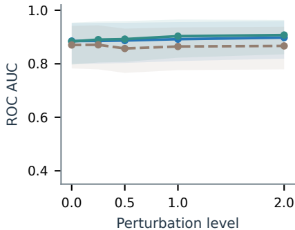
b sEMG
