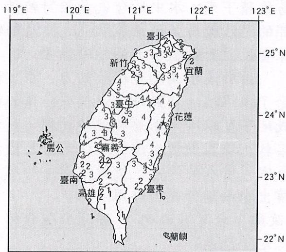
圖說：★表震央位置，阿拉伯數字表示該測站震度
