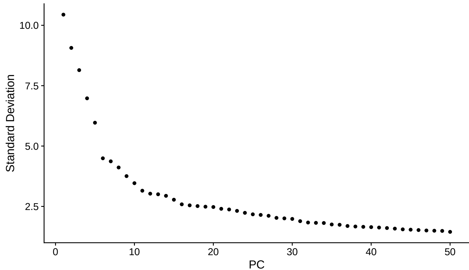
PCA Elbow Plot
