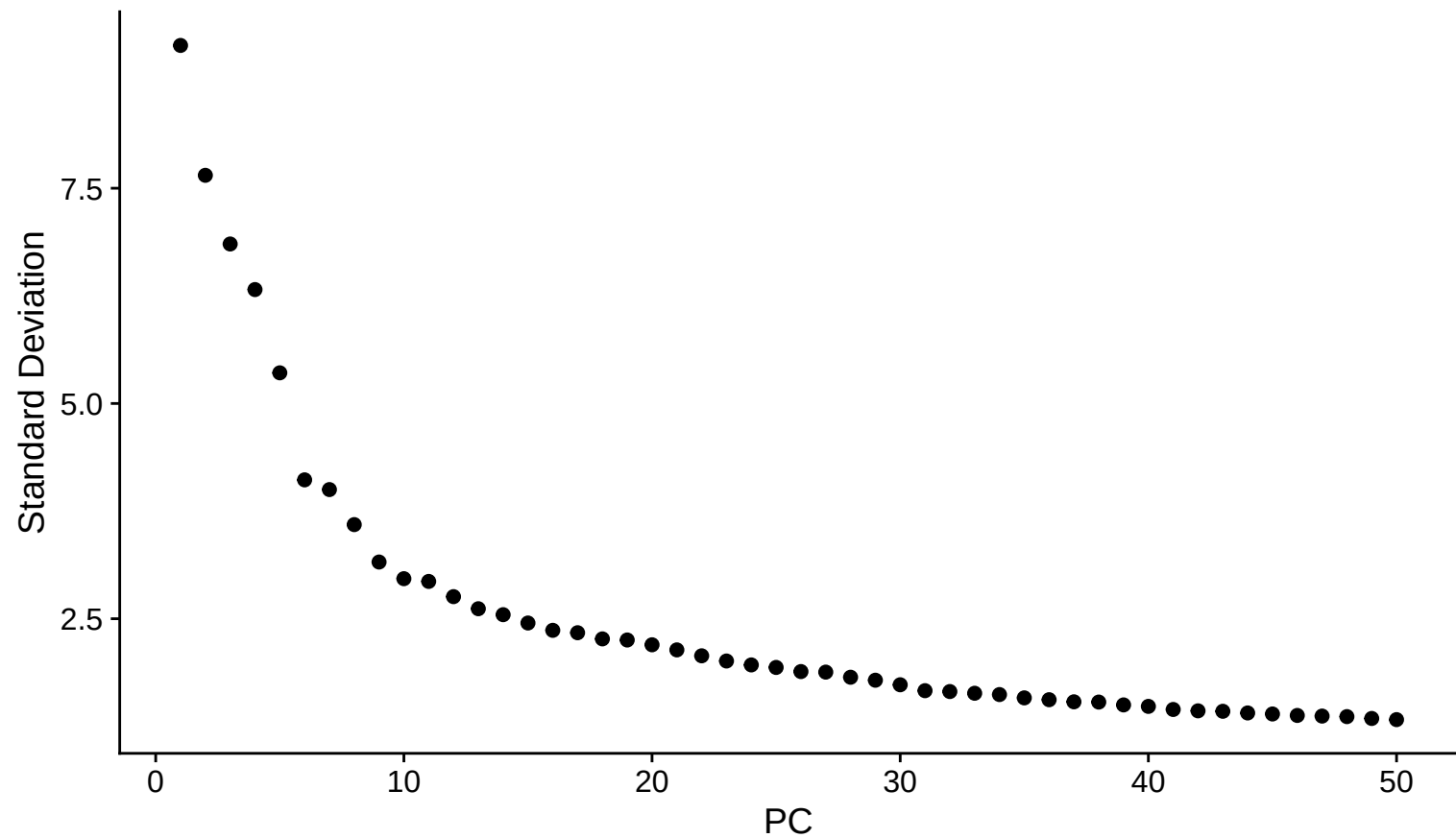
04 PCA Elbow Plot
