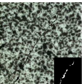
tile-crack
