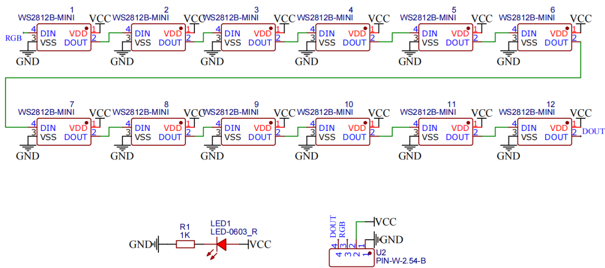
图 8：RGB 灯环原理图
