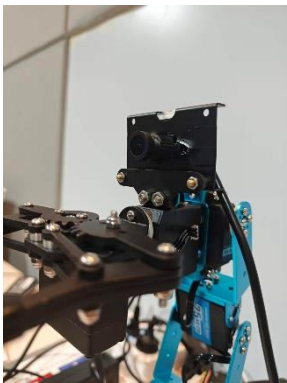
“眼在手上”摄像头 图 9
