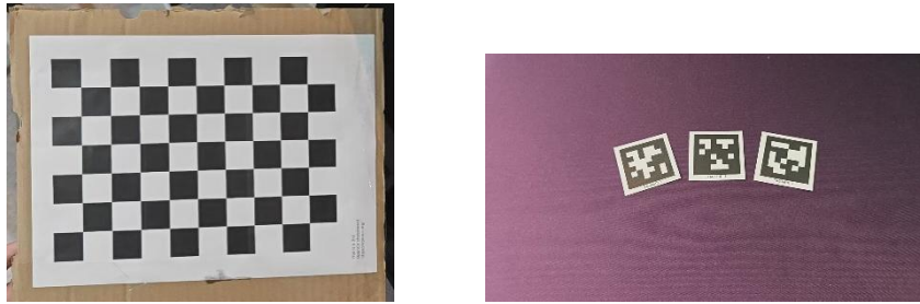
图 12：用于相机标定与手眼标定的棋盘格标定板和 ArUco 标记
