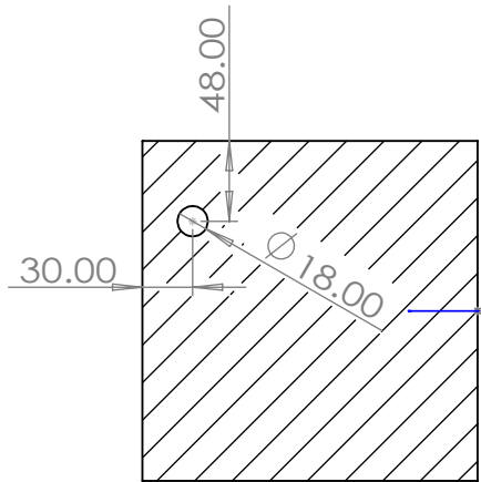
中间隔板
