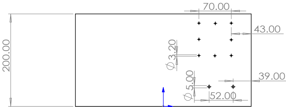
前视图
