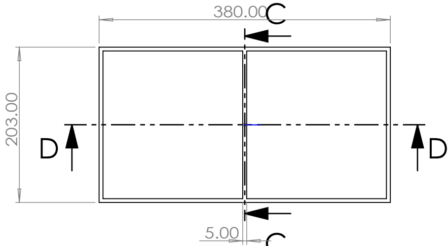
上视图
