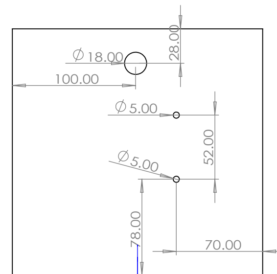
右视图
