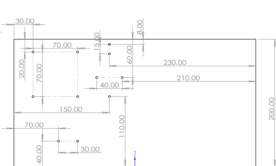
后视图 后视图中的孔直径都是3.2mm
