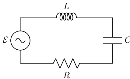
Σχήμα 9.1: Κύκλωμα RLC εναλλασσόμενου ρεύματος
