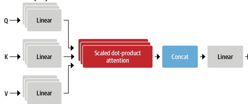
Figura 6 – Diagrama de bloques para un bloque de atención multi-cabeza.
