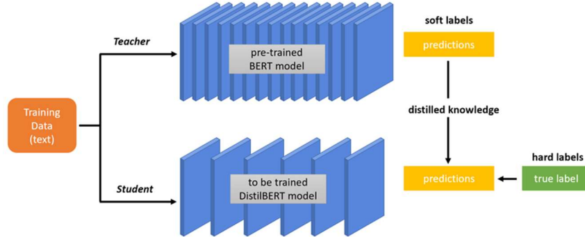
Figura 9 – Esquema de destilado para el entrenamiento de DistilBERT.
