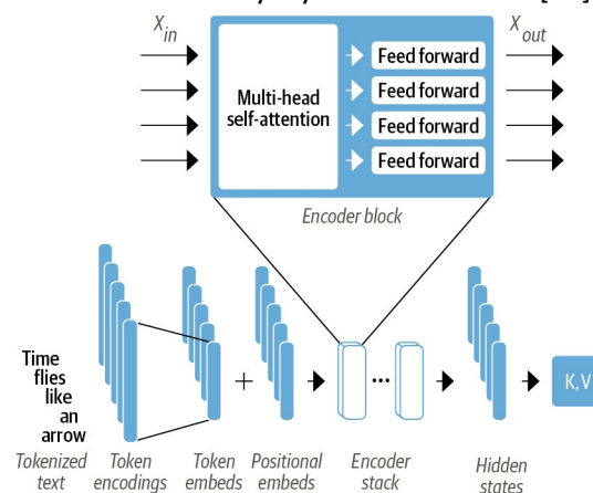
Figura 7 – Esquema Transformer encoder-only con atención multi-cabeza
