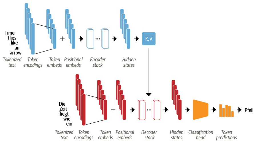
Figura 4 – Esquema de un Transformer encoder-decoder para predicción de tokens.
