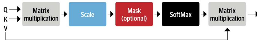
Figura 5 – Diagrama de bloques para una capa de atención.
