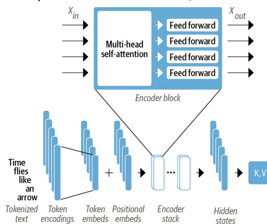
Figura 7 – Esquema Transformer encoder-only con atención multi-cabeza
