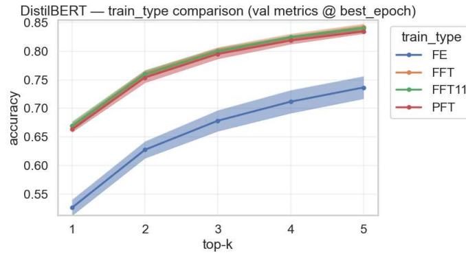
Figura 23 - Rendimiento de los modelos DistilBERT en sus distintos top-k (aciertos en los recomendados) y según el tipo de entrenamiento.
