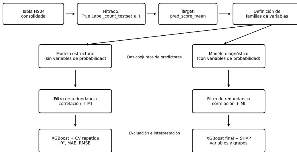
Figura 31 – Diagrama de proceso y análisis de los modelos explicativos del error.
