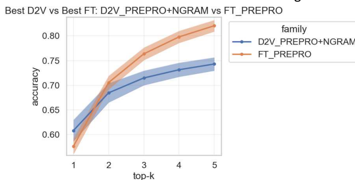
Figura 21 – Comparación de rendimientos de los mejores baselines en sus distintos top-k (aciertos en los recomendados).
