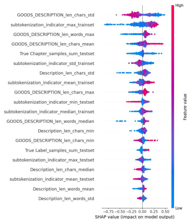
Figura 32 – Visualización beeswarm del shap del modelo estructural.
