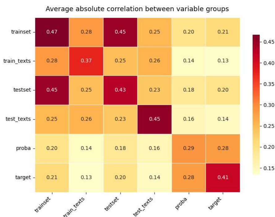
Figura 30 – Matriz de correlaciones medias de features agrupadas según su tipo.
