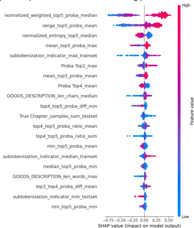
Figura 33 – Visualización beeswarm del shap del modelo diagnóstico.
