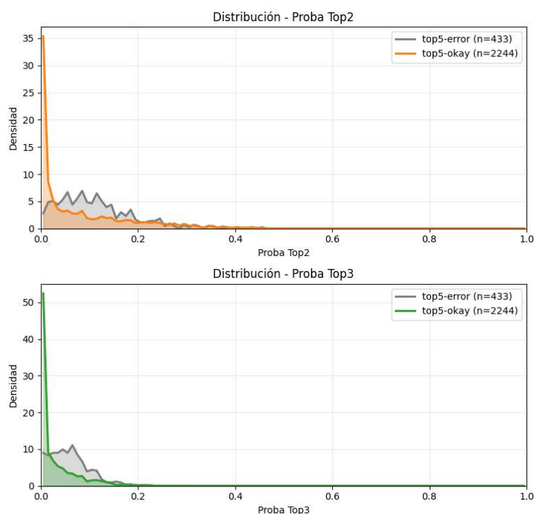
Figura 27 – Distribuciones de Probabilities Top 1 a 3 en la muestra de test.
