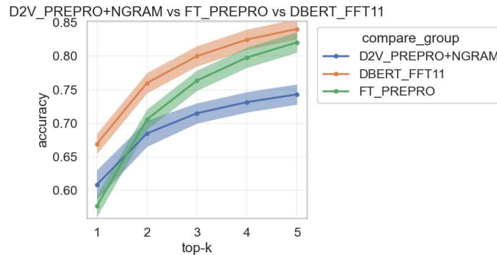
Figura 24 - Comparación de rendimientos de los mejores modelos (baselines y el mejor DistilBERT) en sus distintos top-k (aciertos en los recomendados).
