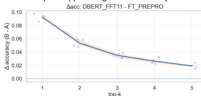
Figura 26 - Gap de rendimiento del mejor DistilBERT vs. el mejor baseline en sus distintos top-k (aciertos en los recomendados).
