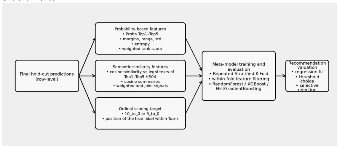
Figura 34 – Proceso de entrenamiento del meta-modelo para evaluación de la clasificación, incluyendo el feature engineering y el test de resultados.
