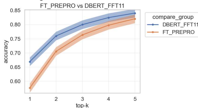
Figura 25 – Comparación de rendimientos de los mejores modelos 1 vs. 1 (mejor baseline y el mejor DistilBERT) en sus distintos top-k (aciertos en los recomendados).
