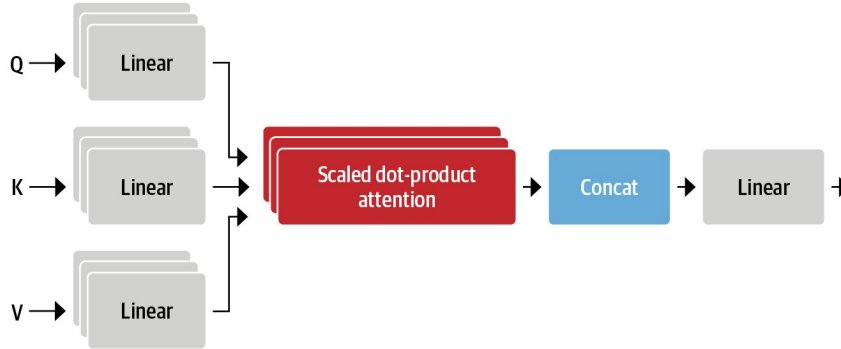
Figura 6 – Diagrama de bloques para un bloque de atención multi-cabeza.
