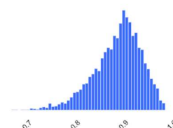
Figura 18 – Estadísticos de la similitud del coseno máximo entre la descripción y el texto legal de la nomenclatura.
