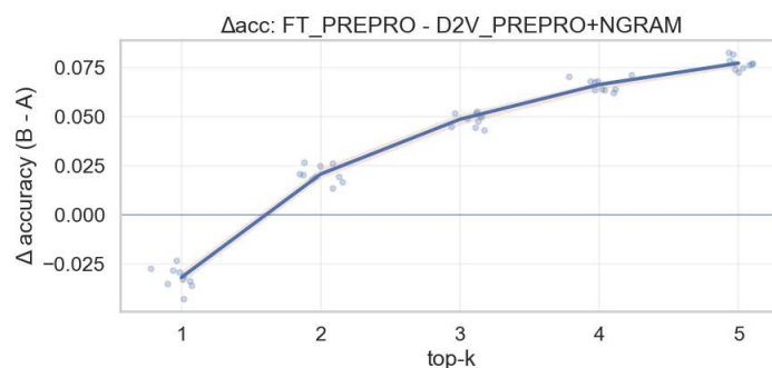
Figura 22 – Gap de rendimiento de los mejores baselines en sus distintos top-k (aciertos en los recomendados).
