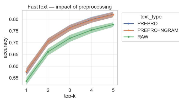
Figura 20 – Rendimiento de los modelos FastText en sus distintos top-k (aciertos en los recomendados) y según el preprocesamiento del input de texto.
