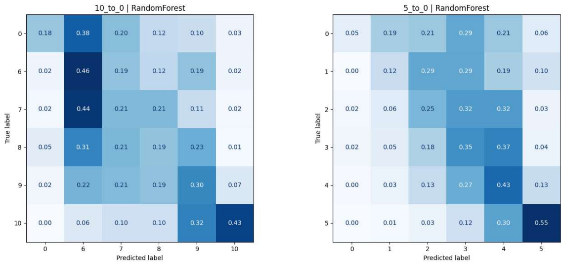
Figura 35 – Matrices de confusión de los meta-modelos, normalizadas por True label.
