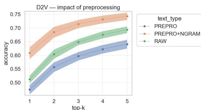
Figura 19 – Rendimiento de los modelos Doc2Vec en sus distintos top-k (aciertos en los recomendados) y según el preprocesamiento del input de texto.
