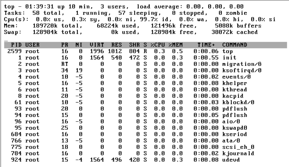
Рис. 5.4. Вывод программы top
