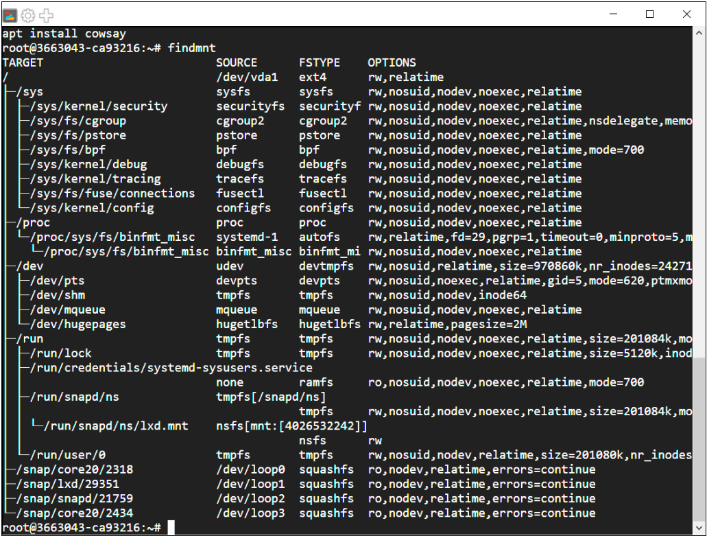
Рис. 4.4. Вывод команды findmnt
