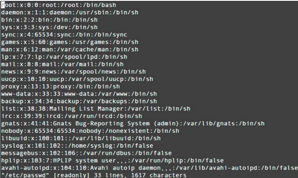
Рис. 8.1. Редактор vi
