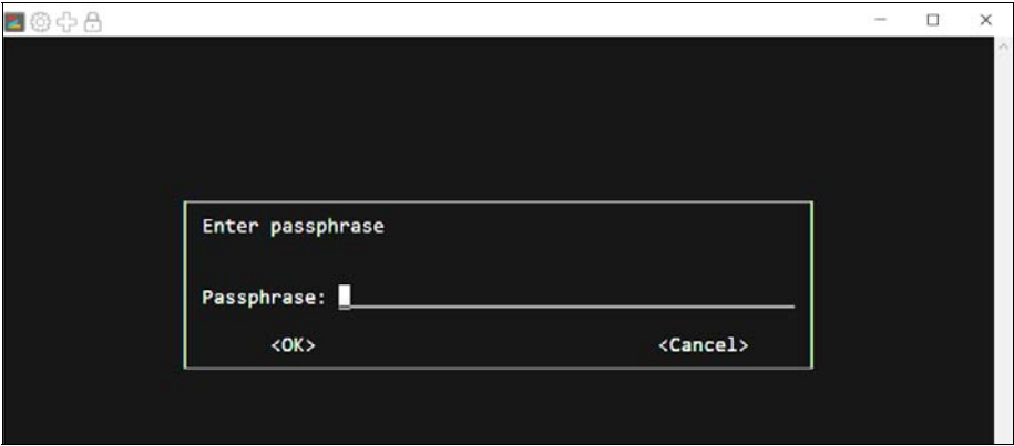
Рис. 8.4. Ввод пароля
