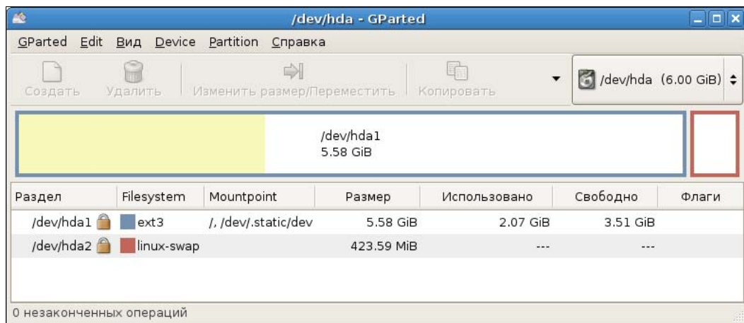
Рис. 11.9. Программа GParted
