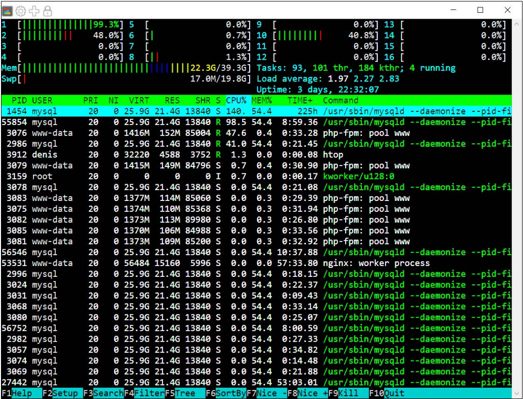
Рис. 5.5. Вывод программы htop
