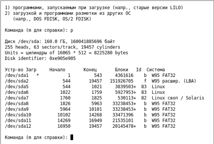
Рис. 4.5. Таблица разделов жесткого диска
