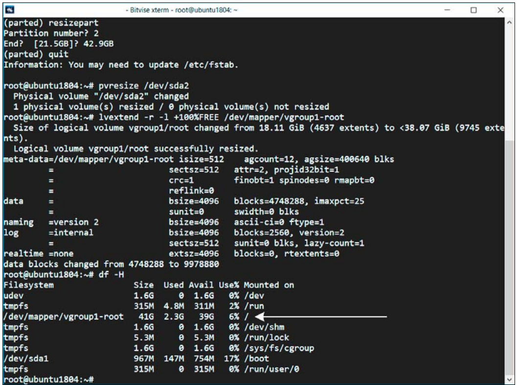
Рис. 11.17. Процедура расширения тома
