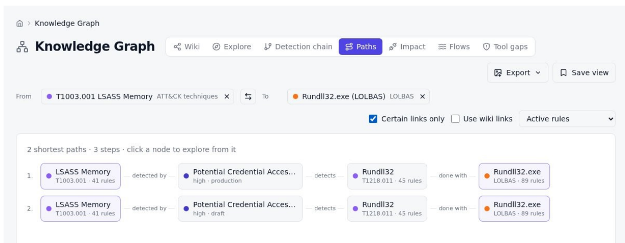
شکل ۳۴ – مسیرهای T1003.001 تا rundll32.exe فقط با ارتباطهای قطعی
