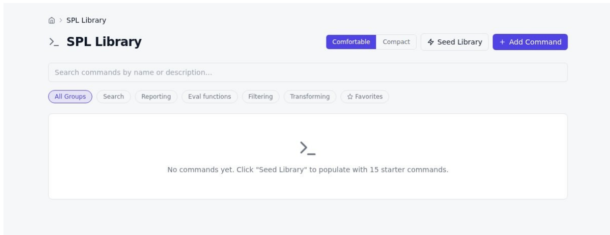
شکل ۳۷ – کتابخانه‌ی SPL
