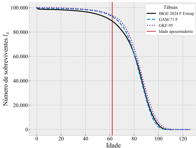
Figura 3 - l_x Feminino
