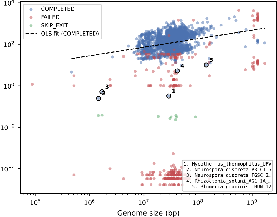
GENEMARK_RUN_SIB (n=1034)
