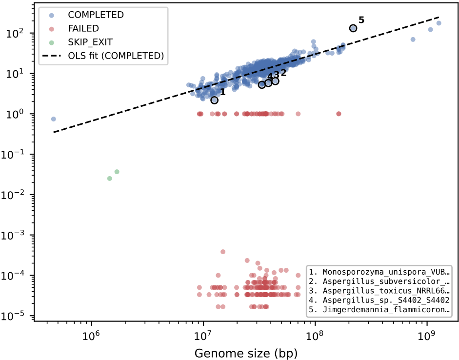
GENEMARK_RUN (n=1357)
