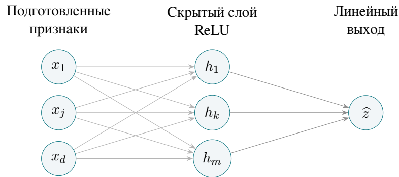
Рис. 1: Схема полносвязной сети. Показаны отдельные компоненты; фактическое число входов определяется после предобработки.
