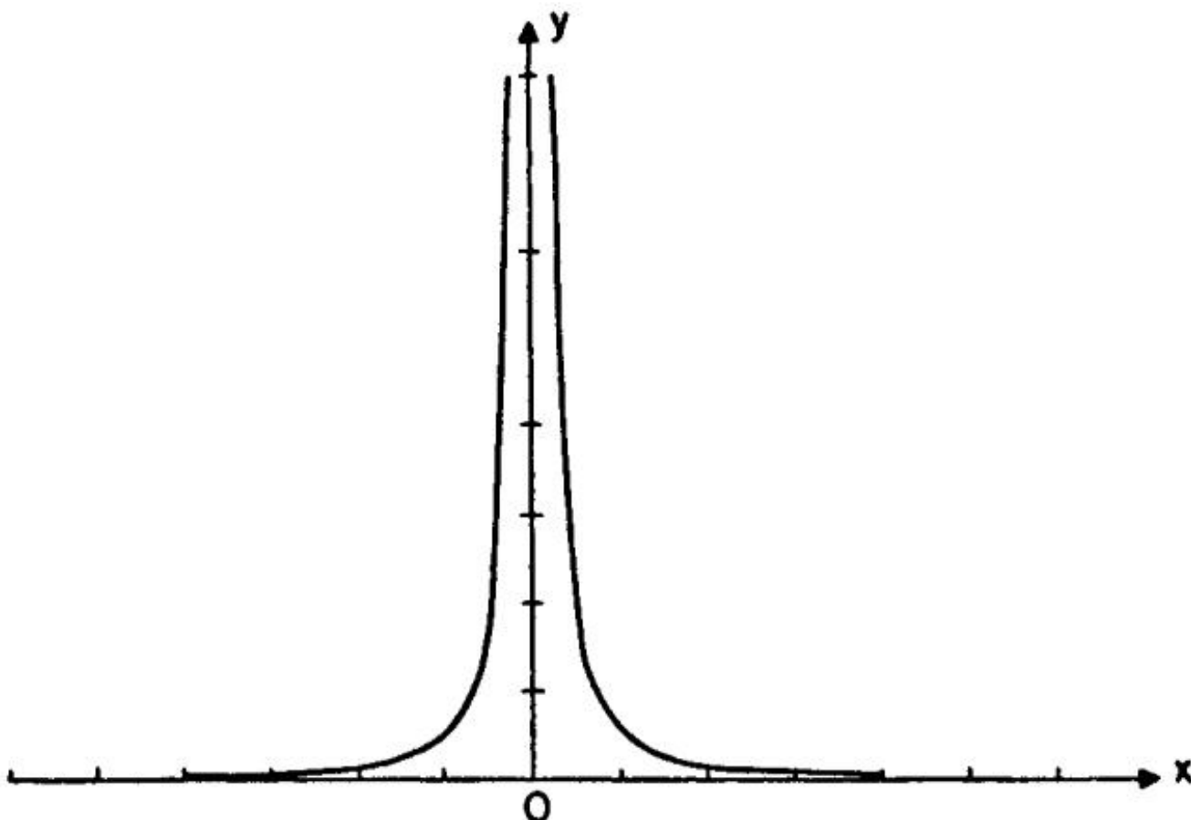
图 35. y = 1/x^2 的图象。
