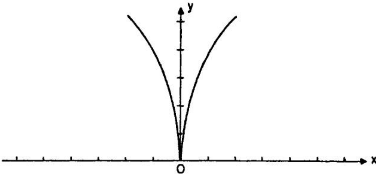
图 36. y = \sqrt[3]{x^2} 的图象。
