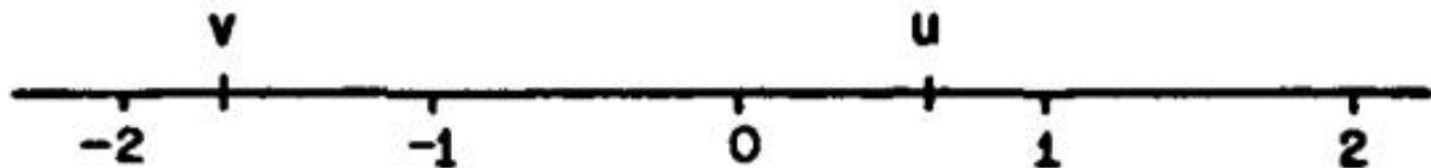
图 18. v < u 的图示
