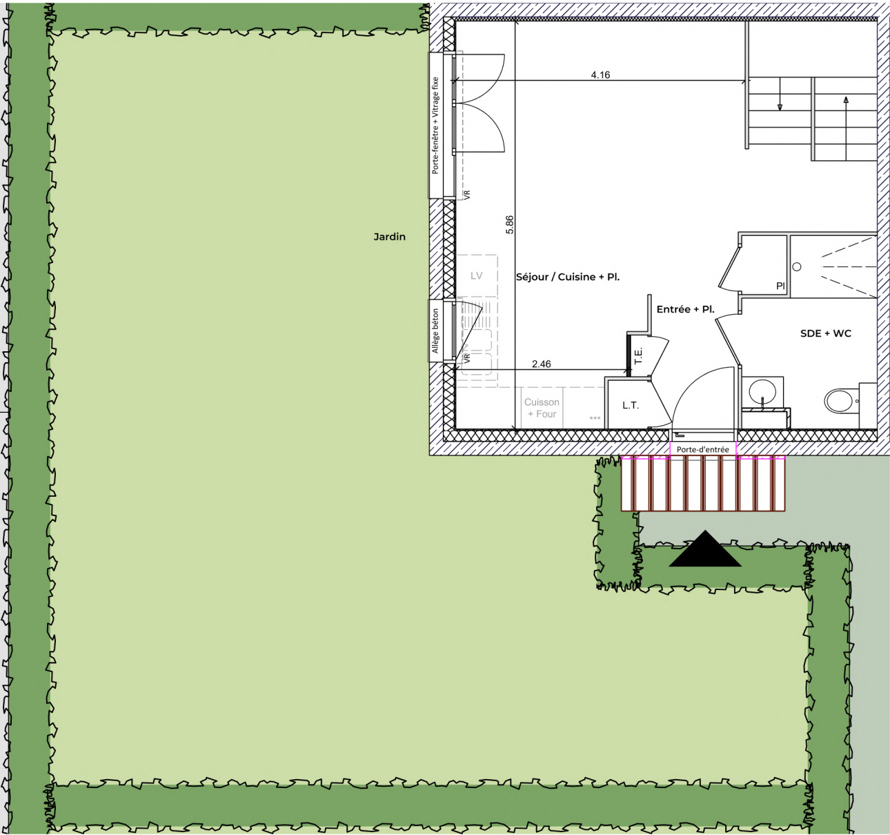
Plan de rez-de-chaussée
