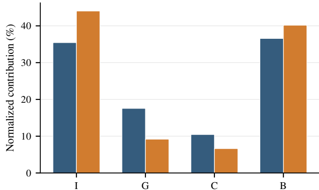
ADNI
