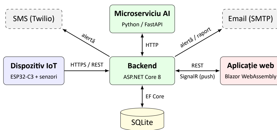
Figura 4: Arhitectura generală a sistemului LifeAlertPlus, cu backend-ul în centru și serviciile externe (Twilio, SMTP) reprezentate prin contururi punctate.
