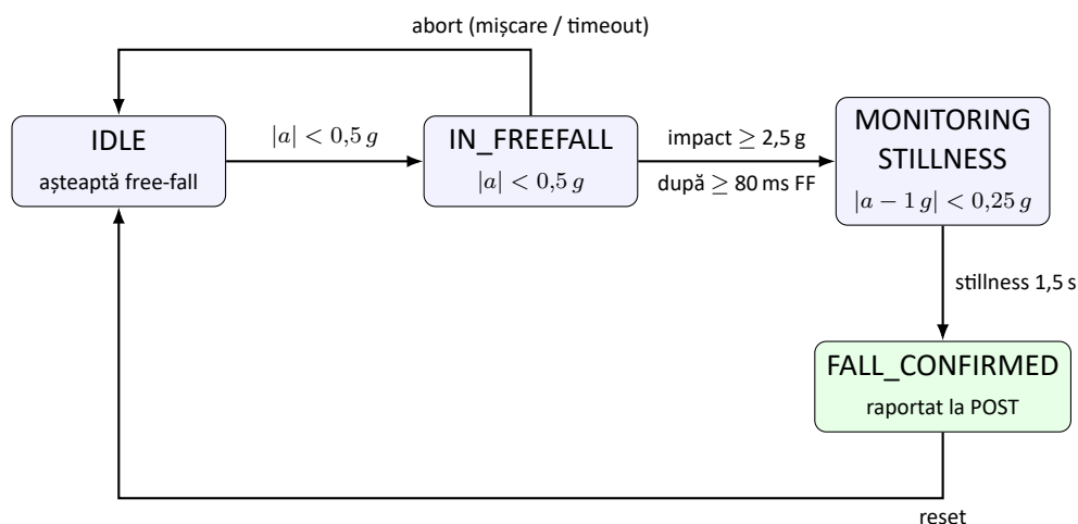
Figura 9: Mașina de stări a detectorului de căderi rulat pe dispozitiv.
