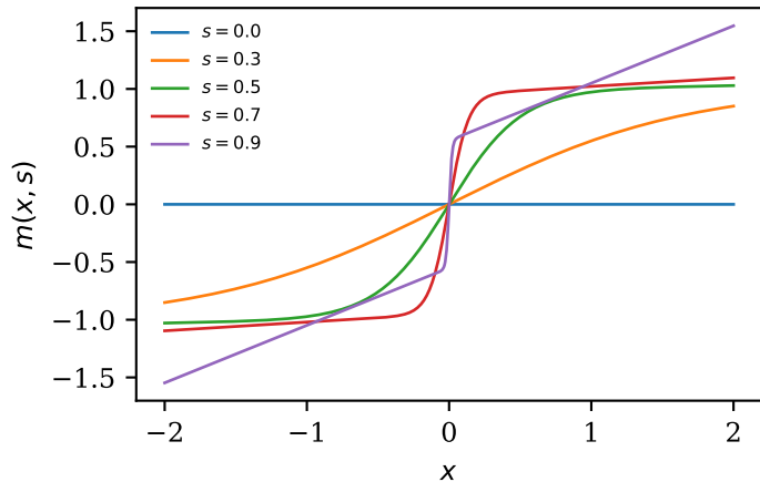
Posterior mean of the endpoint
