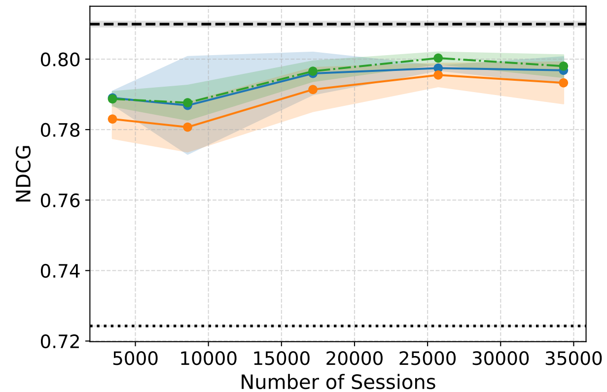
Yahoo!
