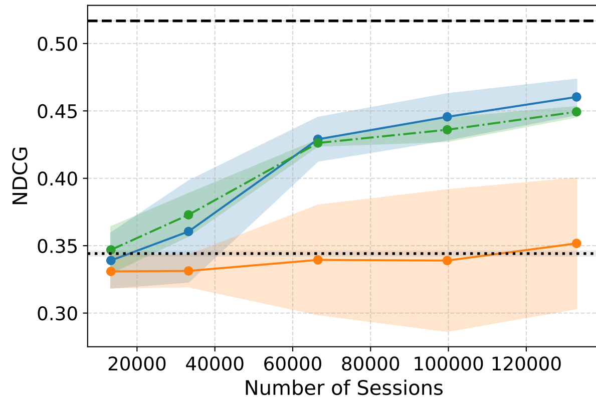
MSLR-WEB30K
