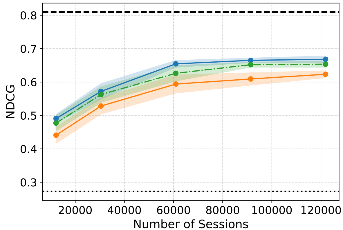
Istella-S
