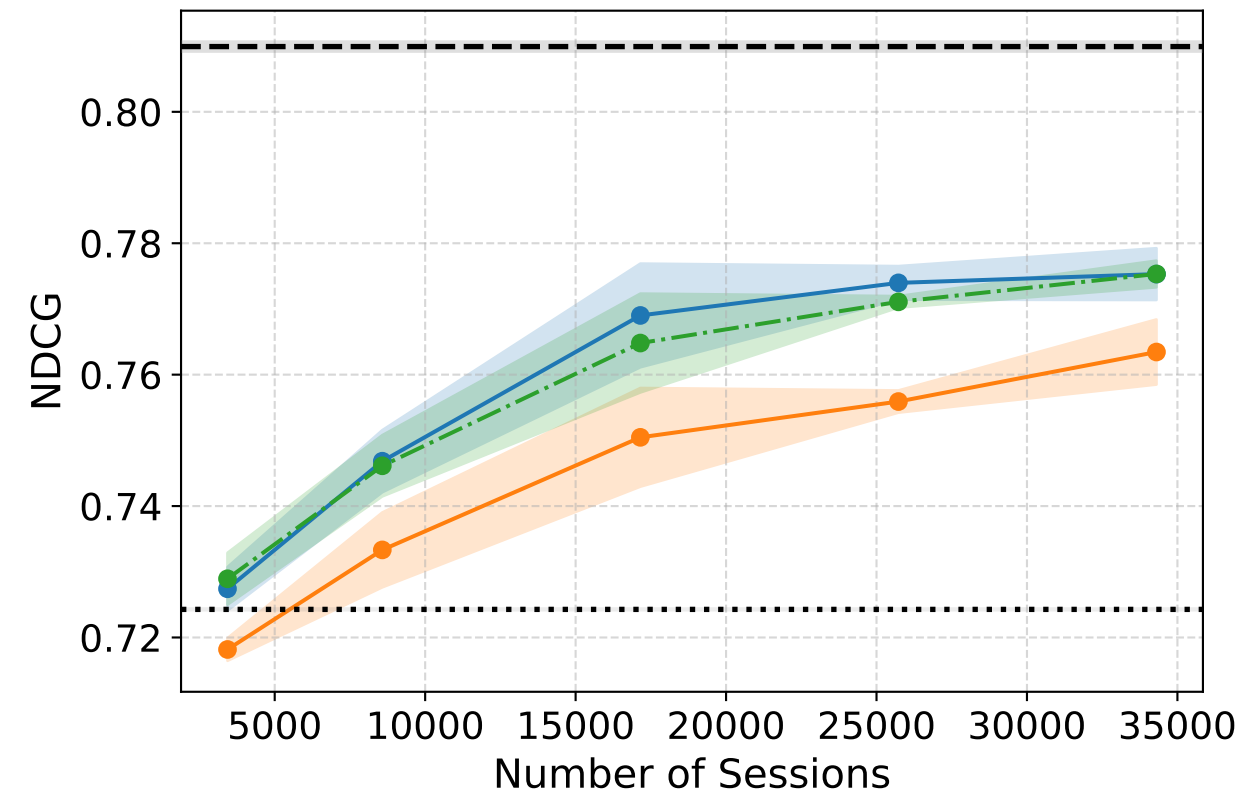
Yahoo!
