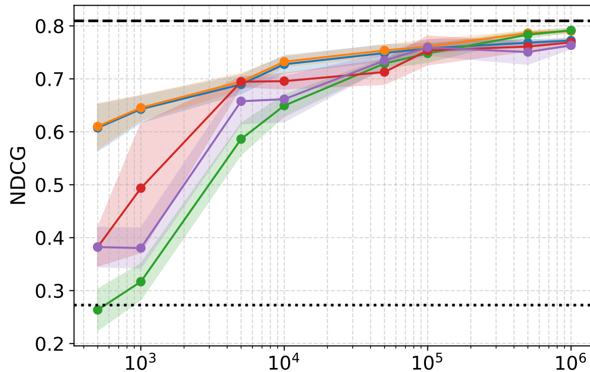
Istella-S
