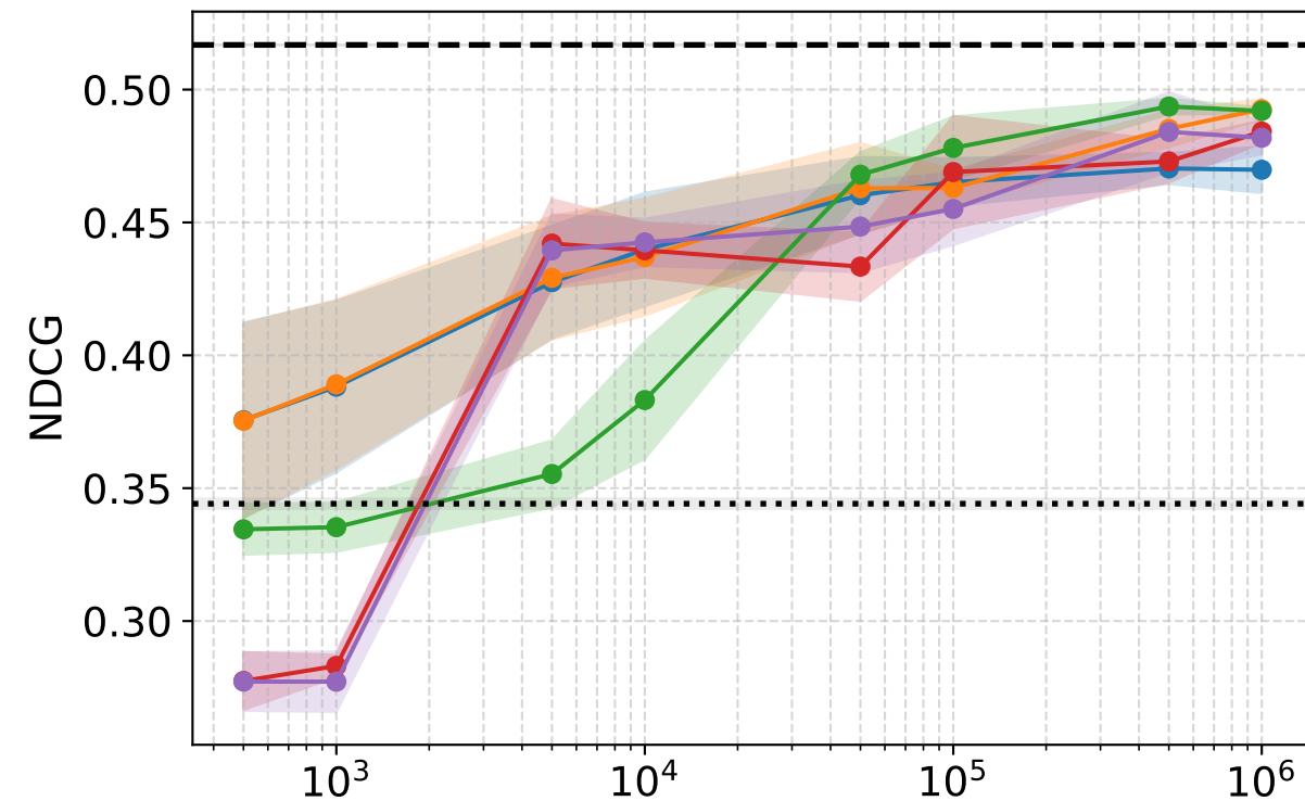
MSLR-WEB30K
