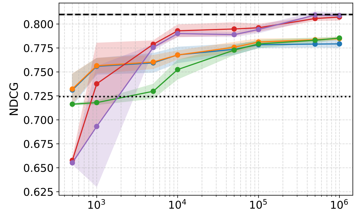
Yahoo!
