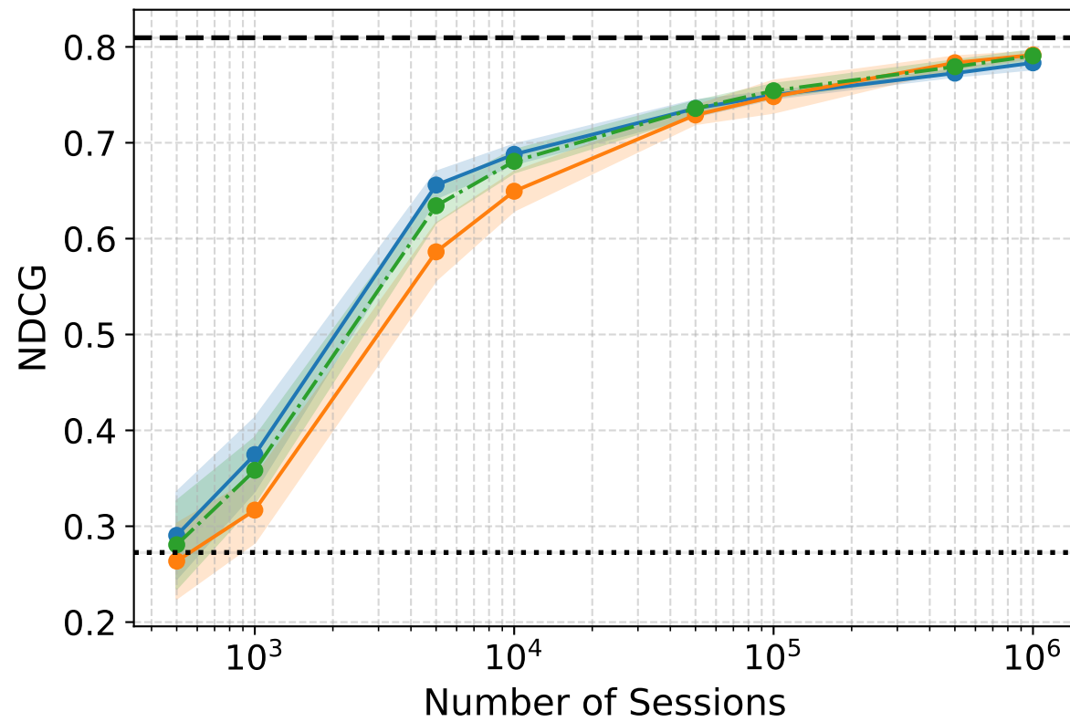
Istella-S
