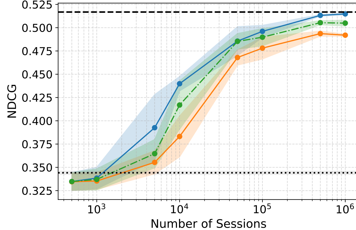
MSLR-WEB30K
