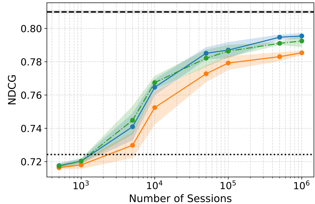
Yahoo!
