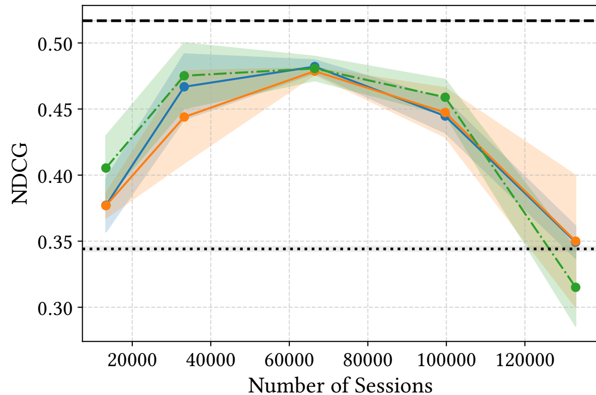
MSLR-WEB30K
