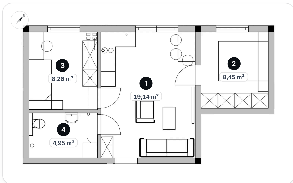
RZUT MIESZKANIA M12
