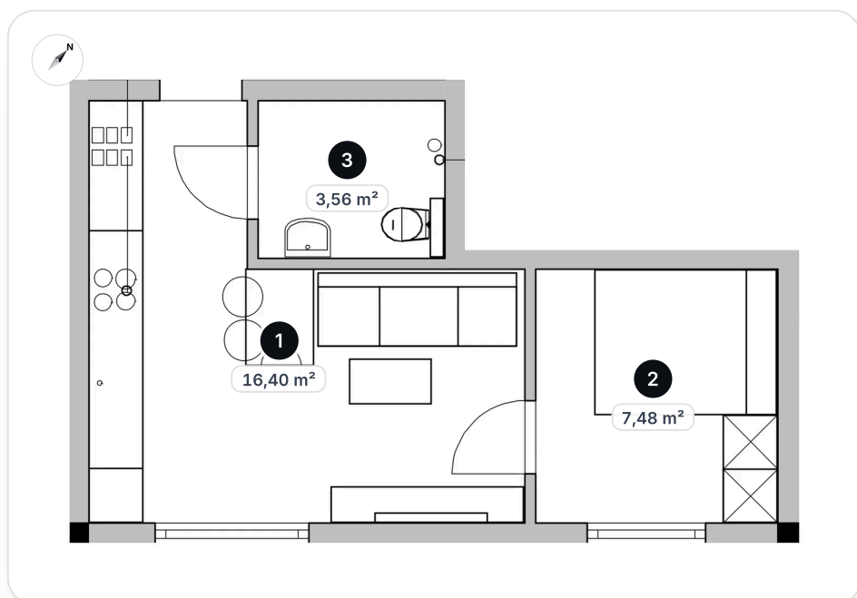
RZUT MIESZKANIA M15
