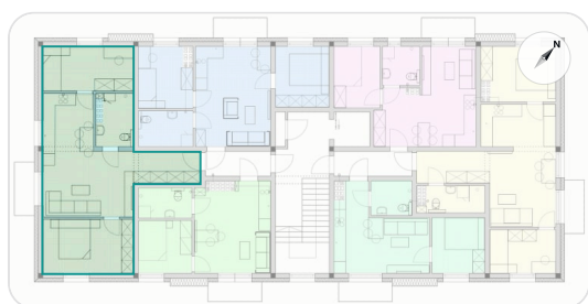
RZUT MIESZKANIA M29
