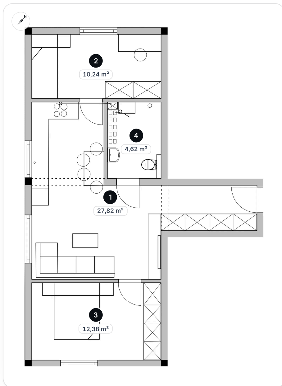
RZUT MIESZKANIA M29
